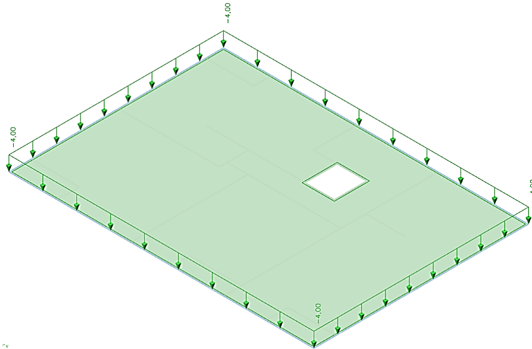
Slika 4.7 Dodatno stalno djelovanje \Delta g ( \text{kN/m}^2 )
