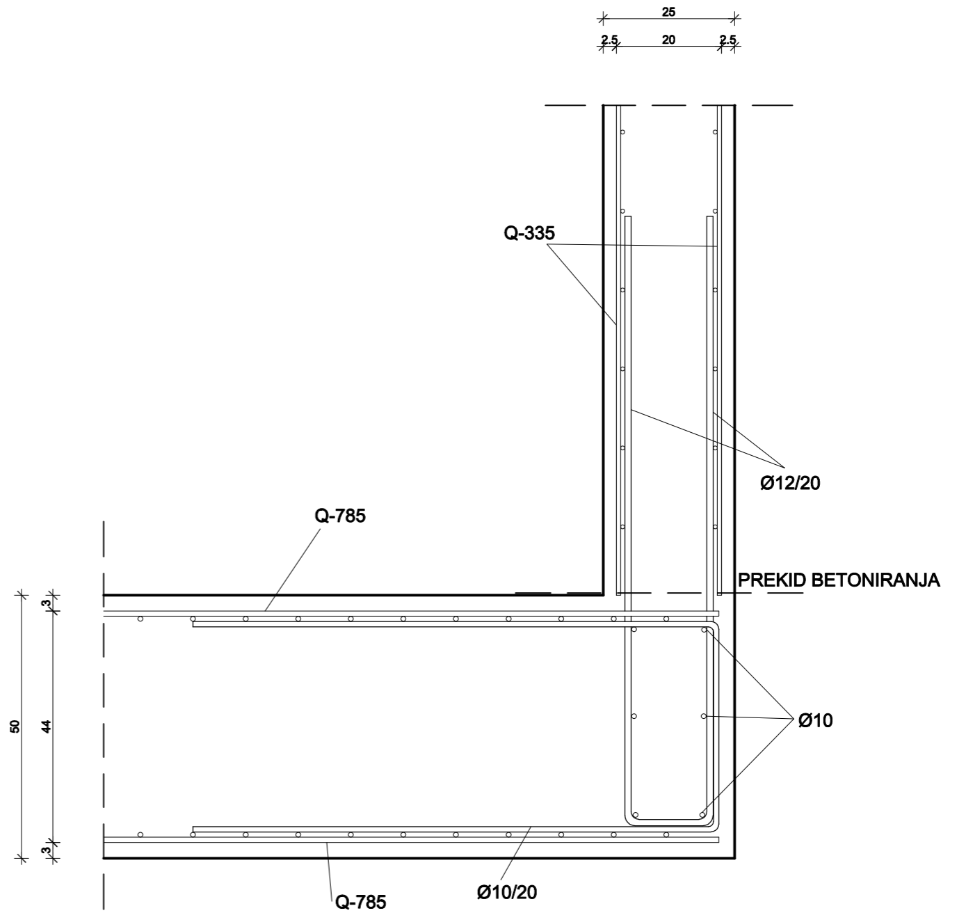
PRESJEK A-A
