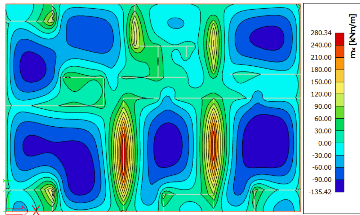
Slika 10.4 Moment savijanja M_{Ed,x} ( \text{kNm/m} ) za GSN-1
