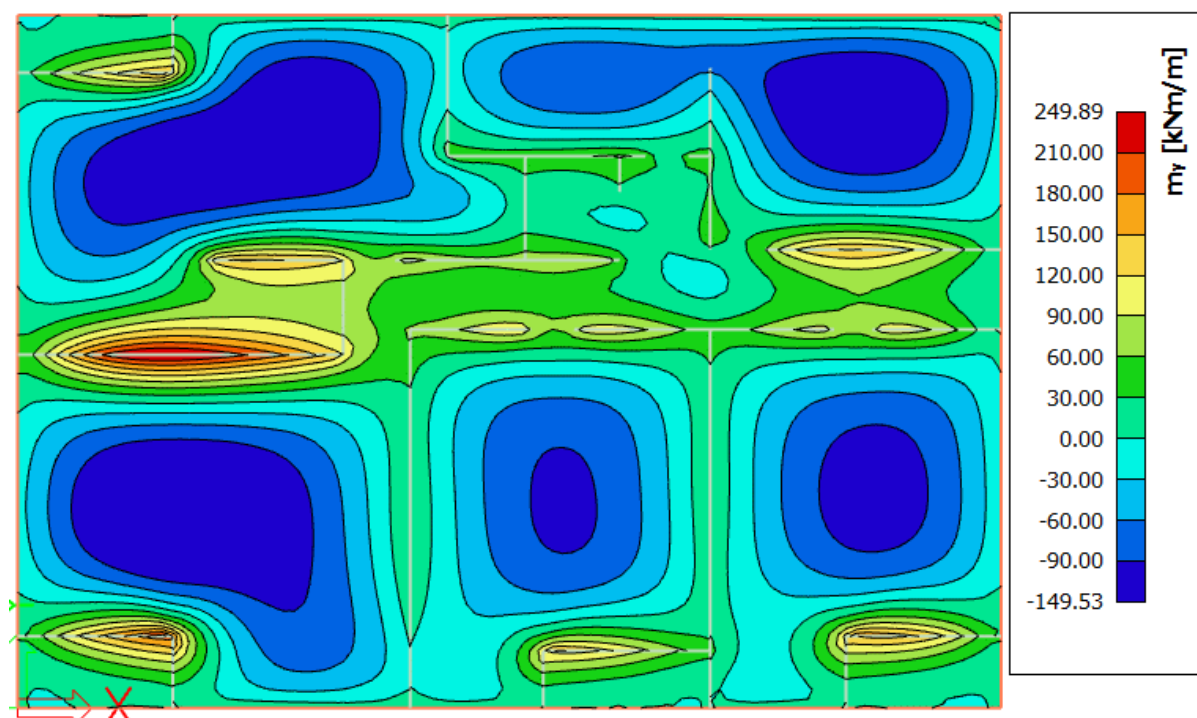
Slika 10.5 Moment savijanja M_{Ed,y} ( \text{kNm/m} ) za GSN-1
