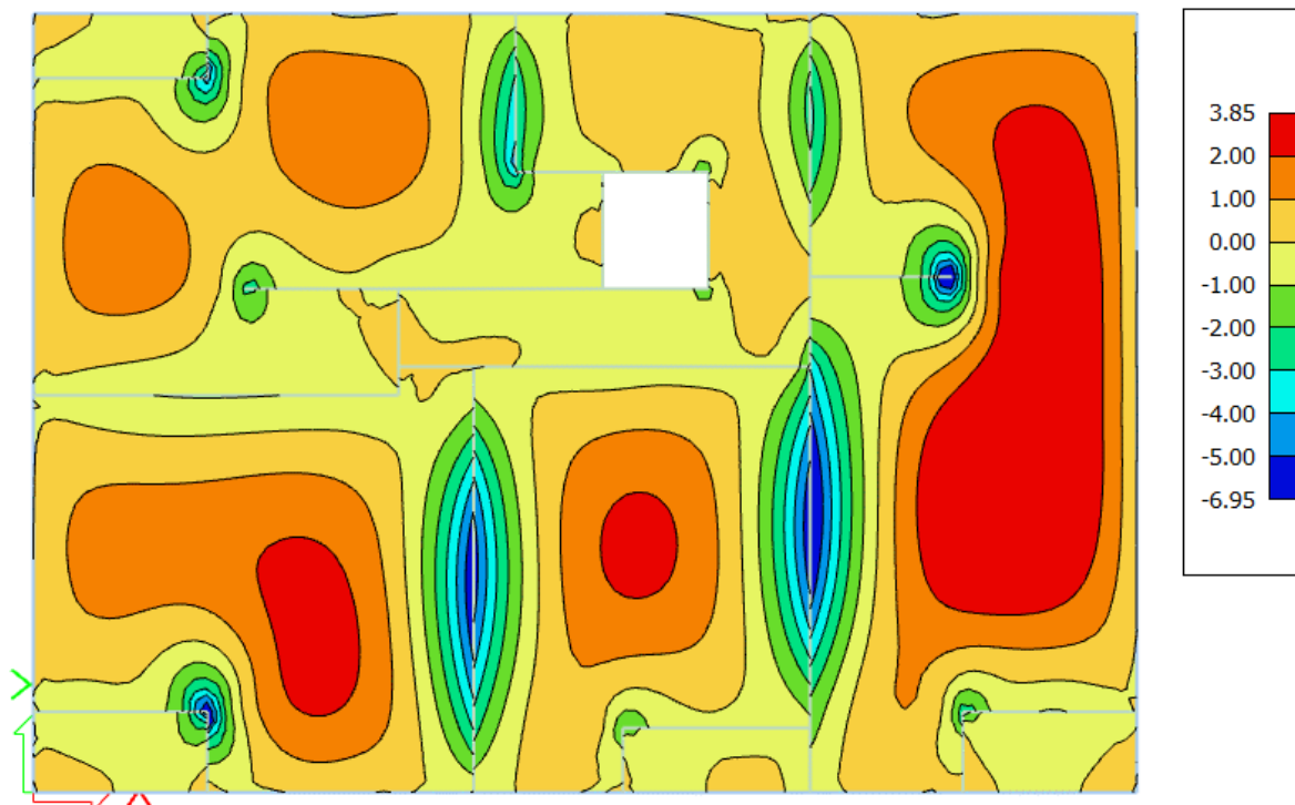
Slika 7.8 Armatura u ploči smjer A_{s,x-x} ( \text{cm}^2/\text{m} ) za GSN-1
