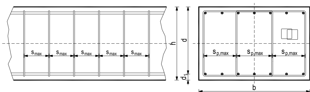
Slika 3.21 – Razmaci spona
