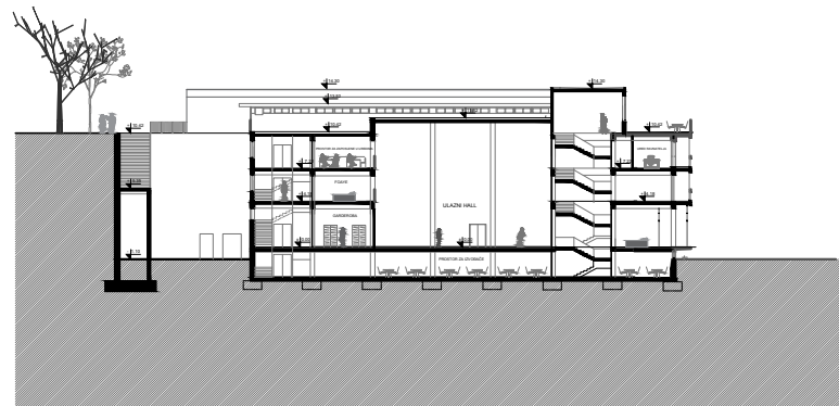
PRESJEK 3 - 3
