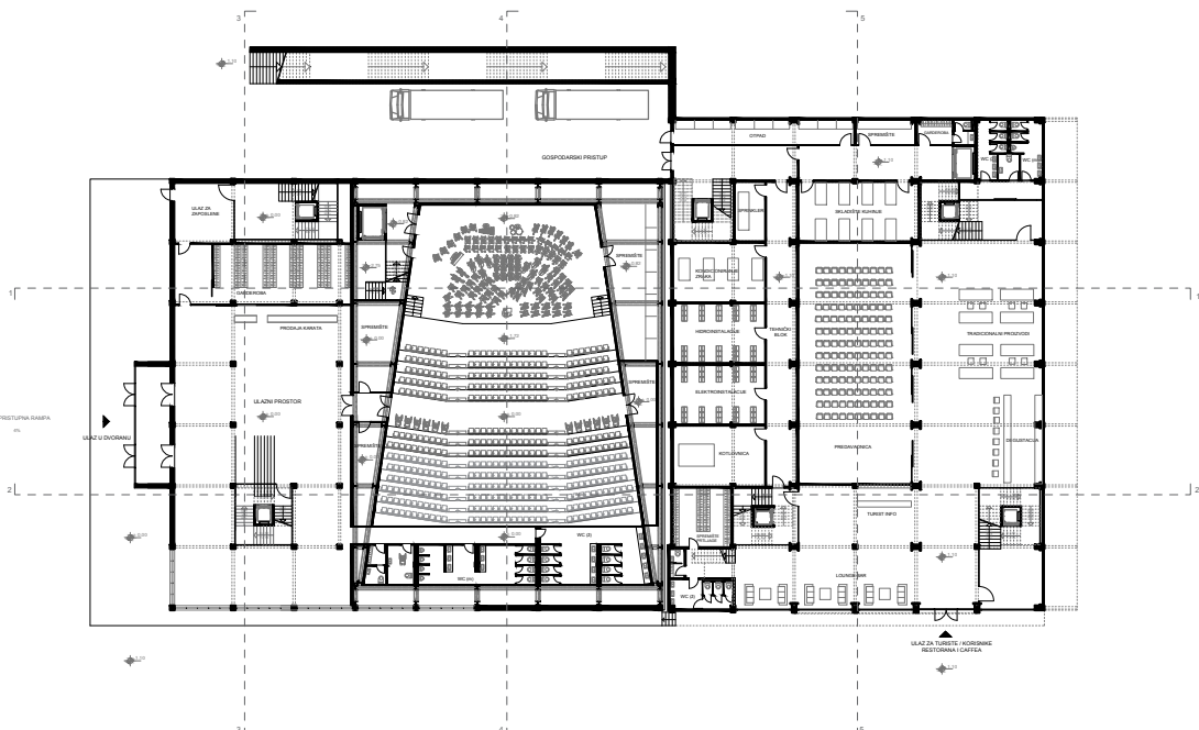
PRIZEMLJE
