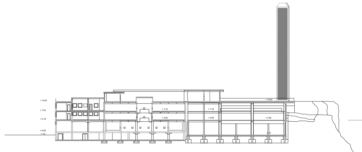
PRESJEK D
