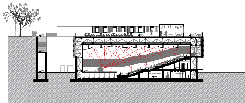
PRESJEK 4 - 4
