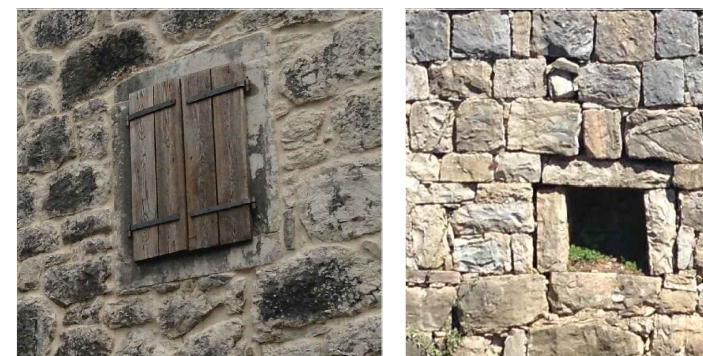
Grafički prilog 59. Prozor sa škurama, Kostanje; nepravilno klesani nadvoji nad prozorima, Gata / fotografije autora analize
