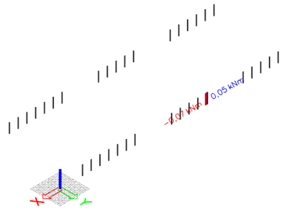
Slika 7.6.3. Moment M_x
