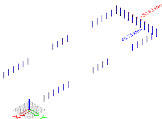
Slika 7.5.3.Moment M_x
