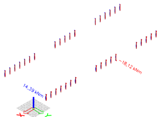
Slika 7.6.5. Moment M_z
