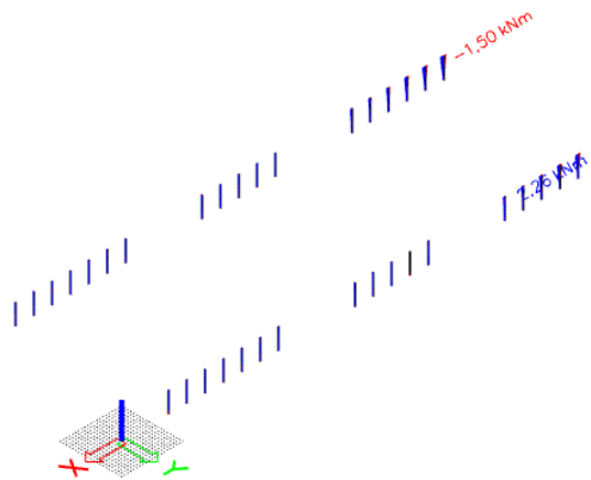
Slika 7.6.3. Moment M_x
