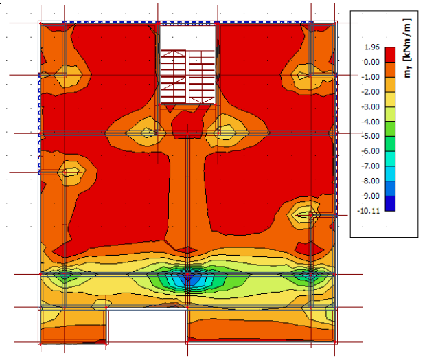
Slika 104 2D dijagram momenata savijanja M_y Dodatno stalno
