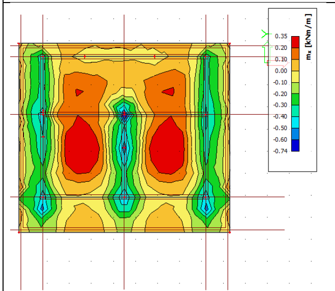
Slika 53 2D dijagram momenata savijanja M_x Vjetar dolje
