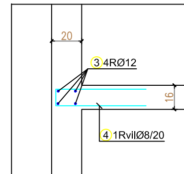
PRESJEK
