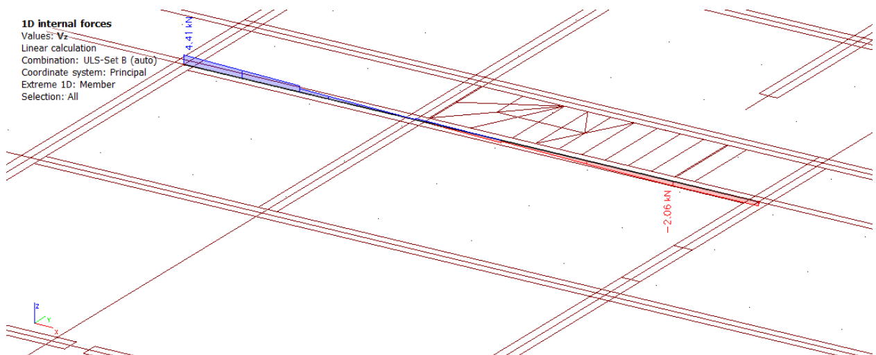
Slika 84 Dijagram poprečnih sila Vz na gredama
