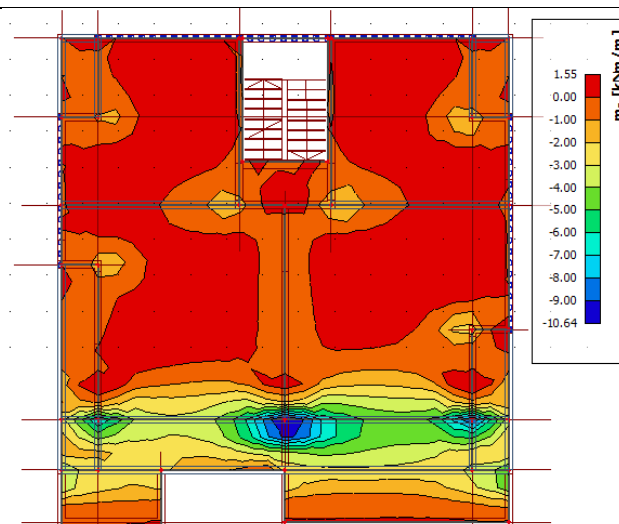
Slika 106 2D dijagram momenata savijanja M_y Promjenjivo
