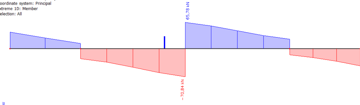
Slika 78 Dijagram poprečnih sila V_z na gredama
