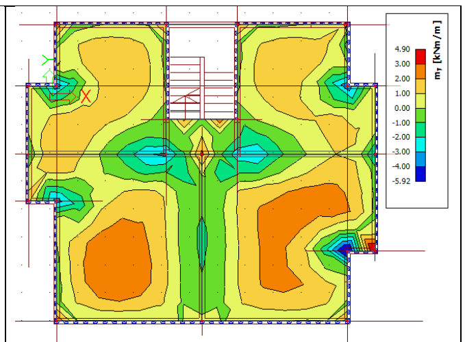
Slika 117 2D dijagram momenata savijanja M_y Vlastita težina
