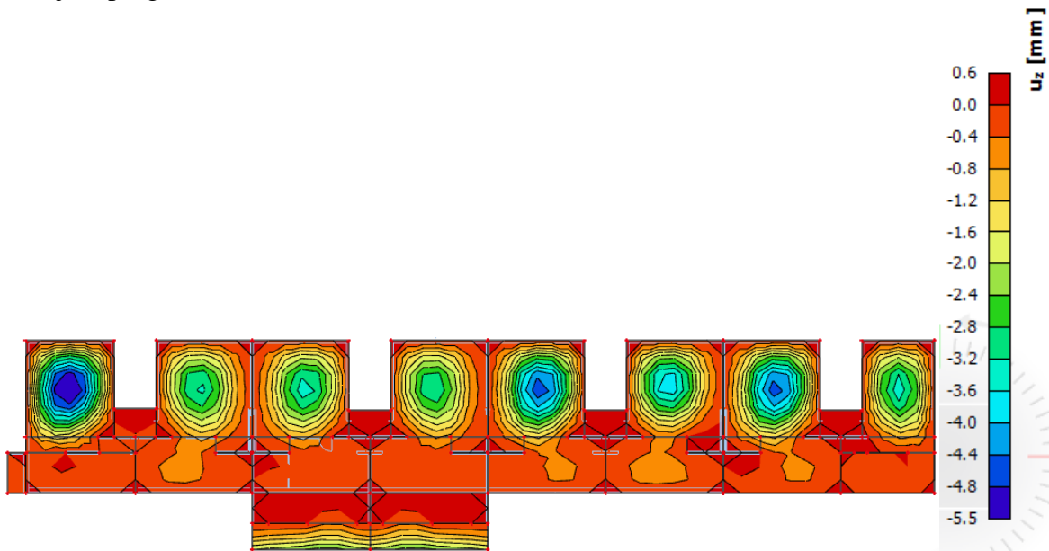
Slika 11.16. Prikaz progiba
