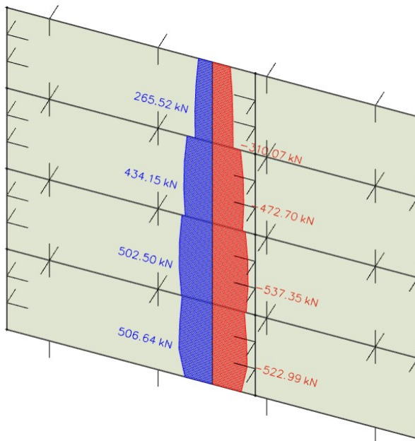
Slika 13.15 Poprečna sila V
