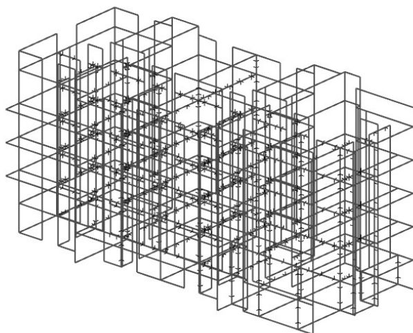
Slika 9.2 Model za proračun – aksonometrija
