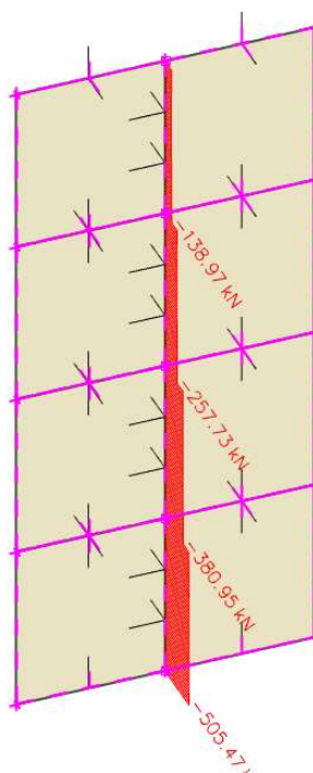
Slika 13.4 Uzdužna sila N
