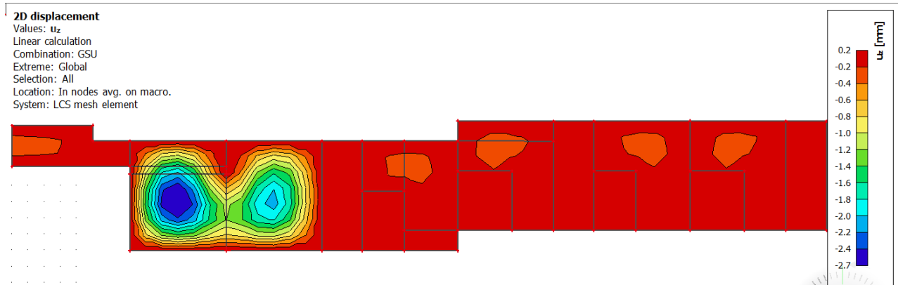
Slika 10.8 Prikaz progiba ploče za kombinaciju GSU
