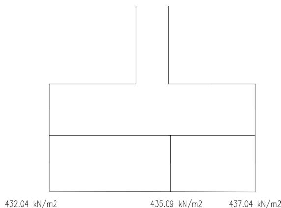
Slika 14.3 Prikaz naprežanja
