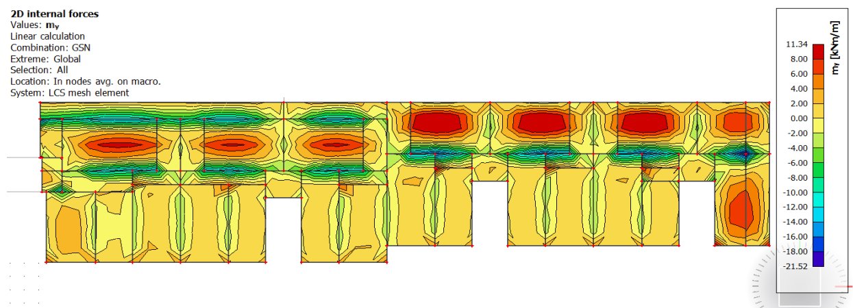
Slika 10.17 Prikaz momenata savijanja (GSN, m_y )
