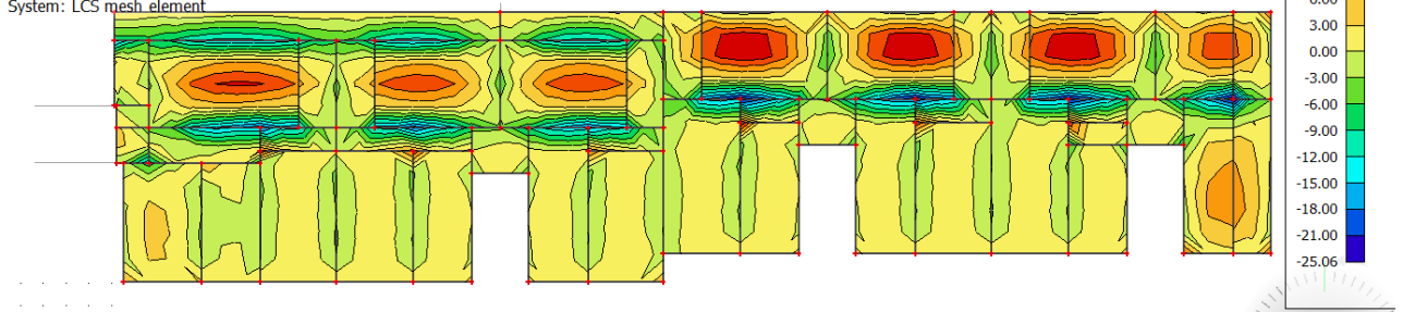
Slika 10.9 Prikaz momenata savijanja (GSN, m_y )
