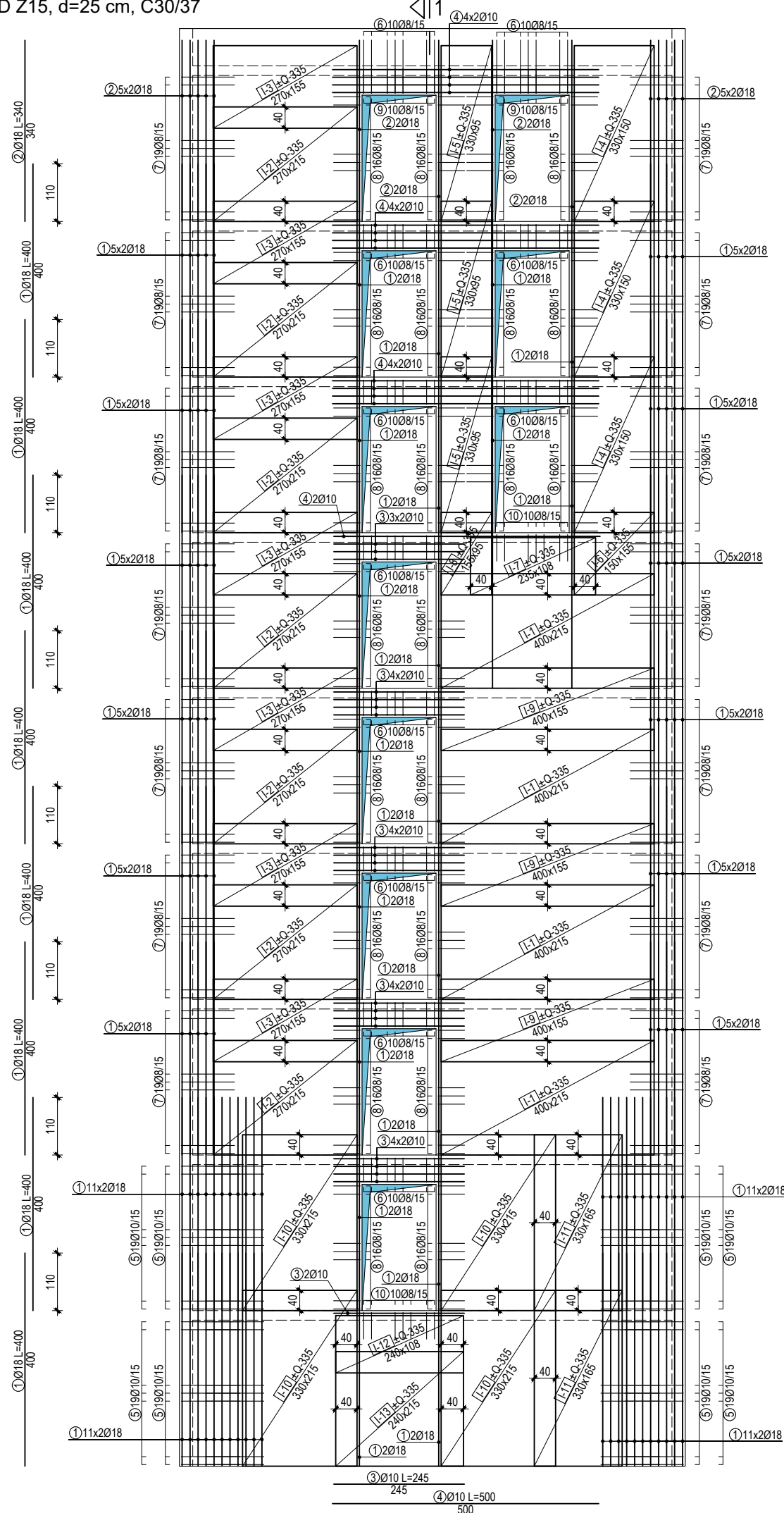
-presjek 1-1, M 1:100
