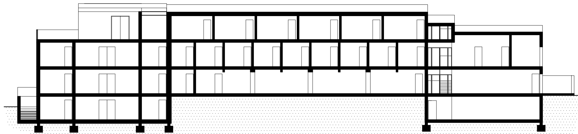
PRESJEK A
