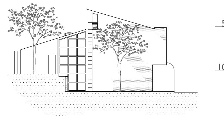
pročelje ISTOK
