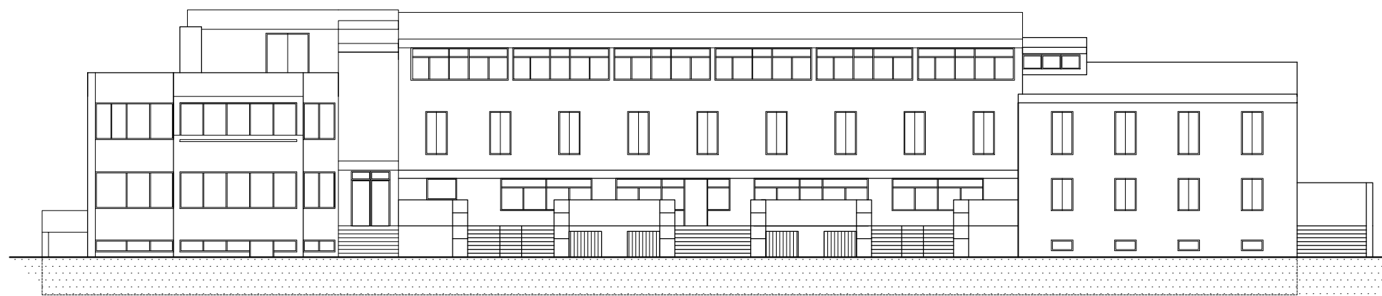
JUŽNO PROČELJE
