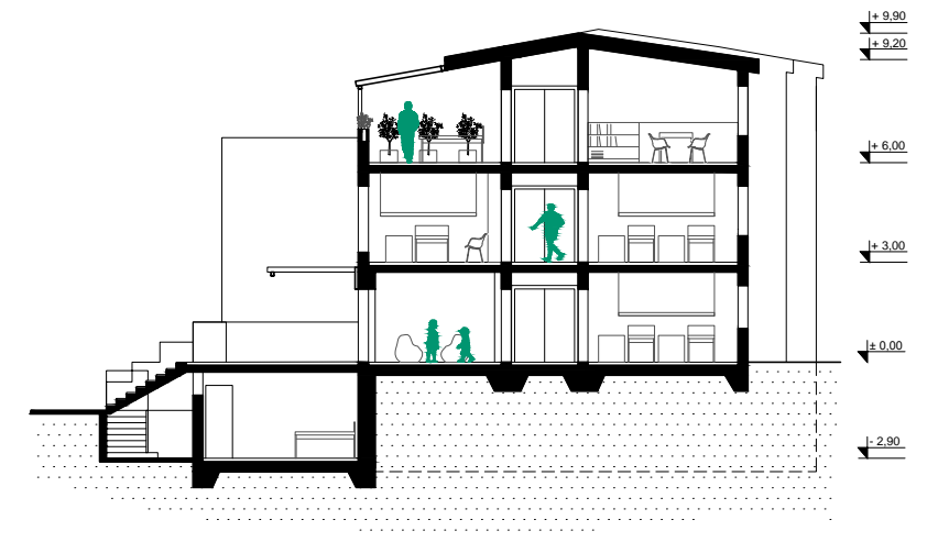
presjek C
