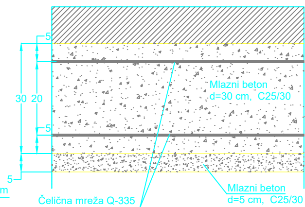
PRESJEK KROZ PODNOŽNI SVOD
