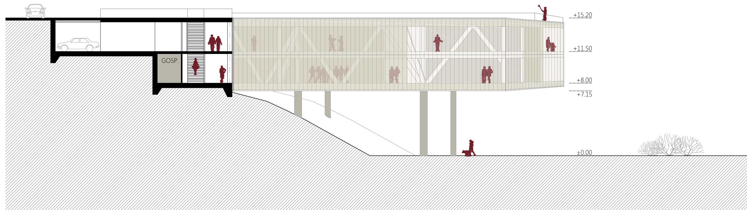
PRESJEK 6-6 M 1:250
