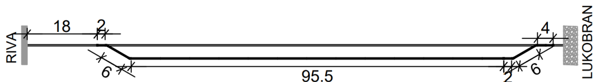
Slika 13. Nacrt cjevovoda
