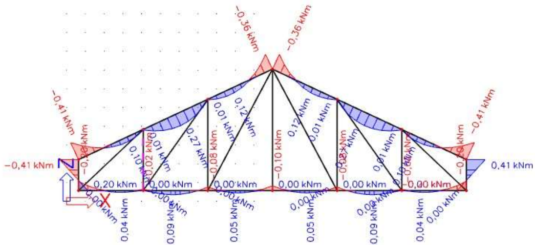
3.9. Momentni dijagram M za GSN 3
