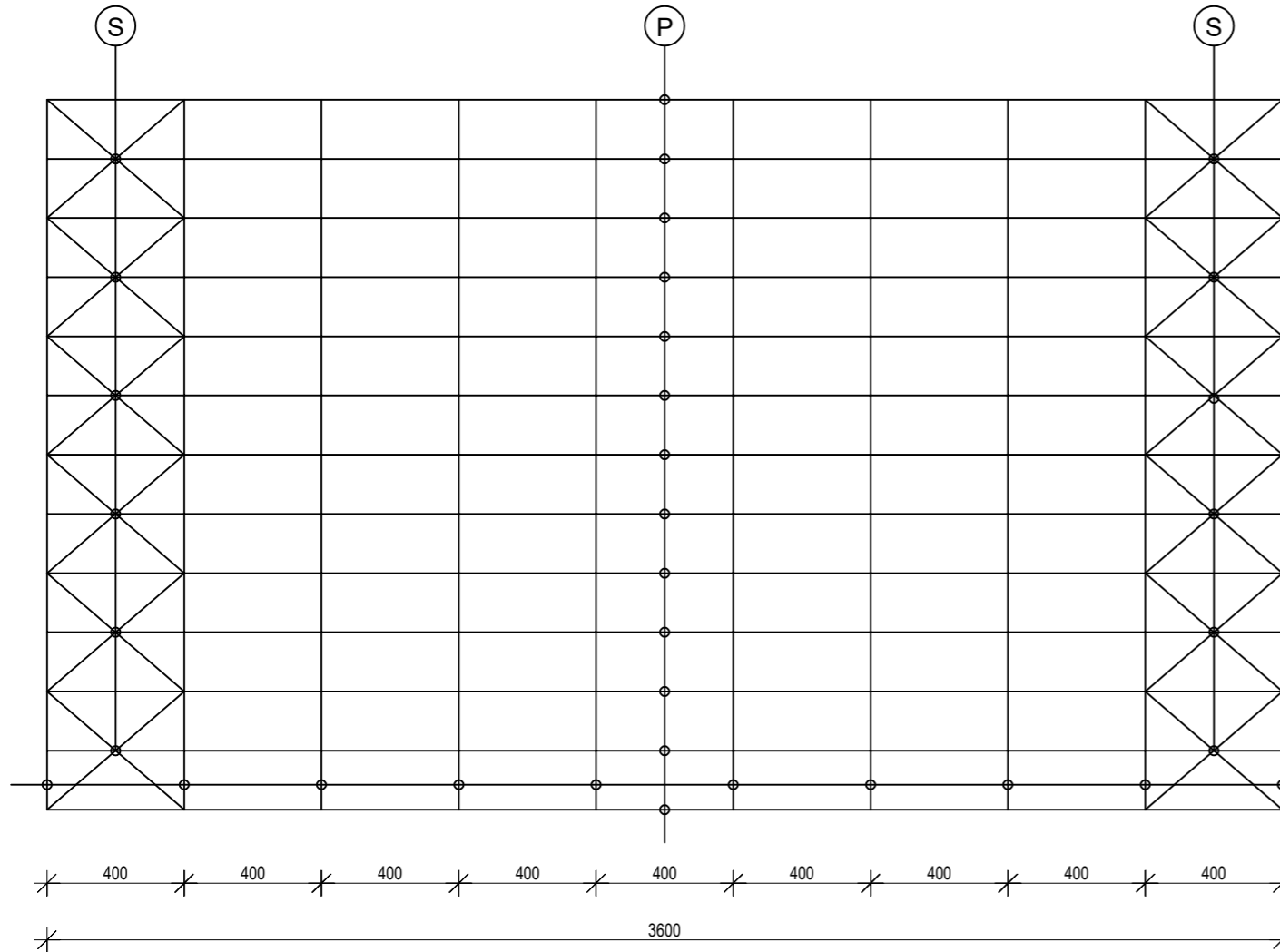
TLOCRT
