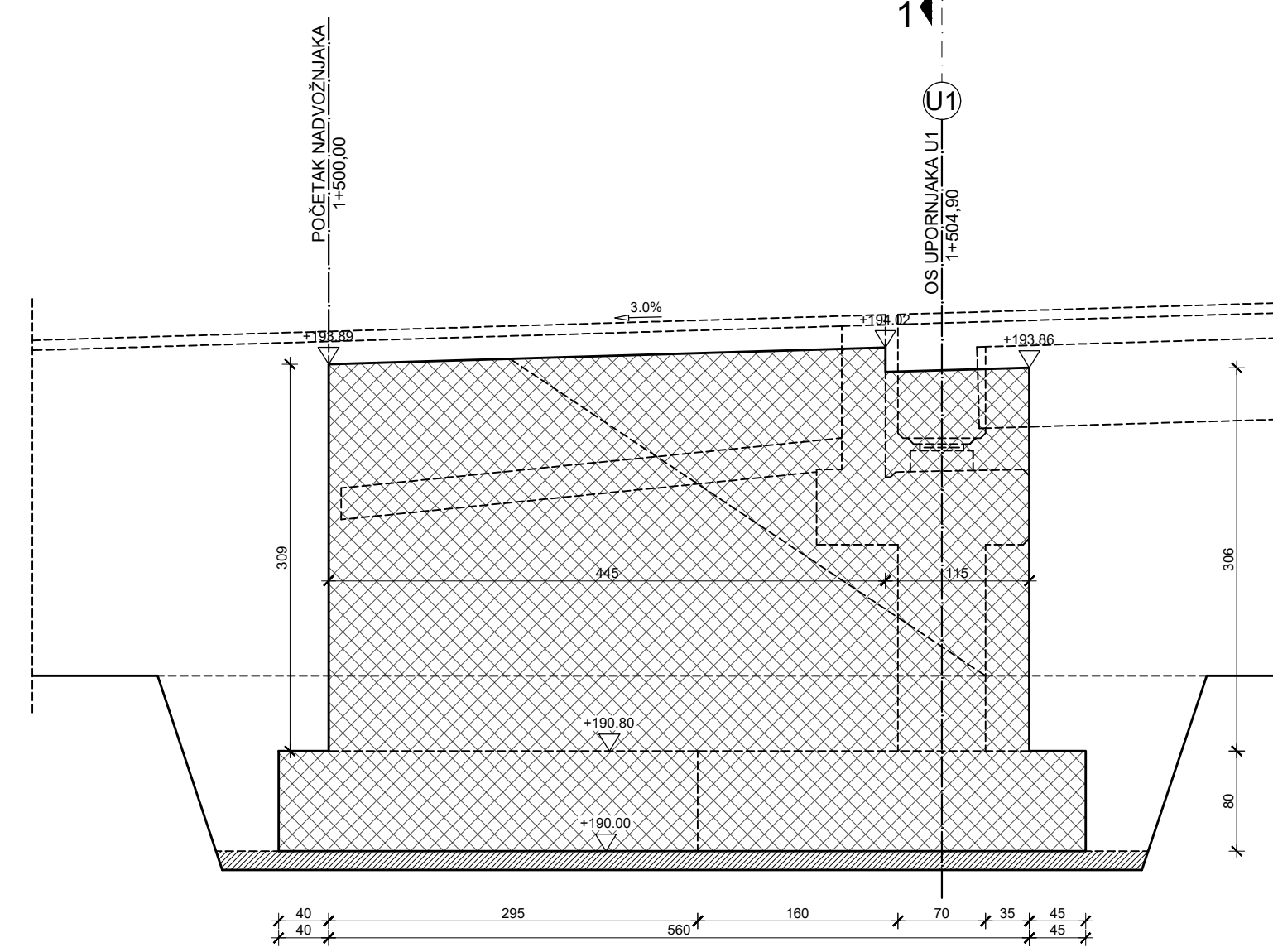
PRESJEK 5-5
