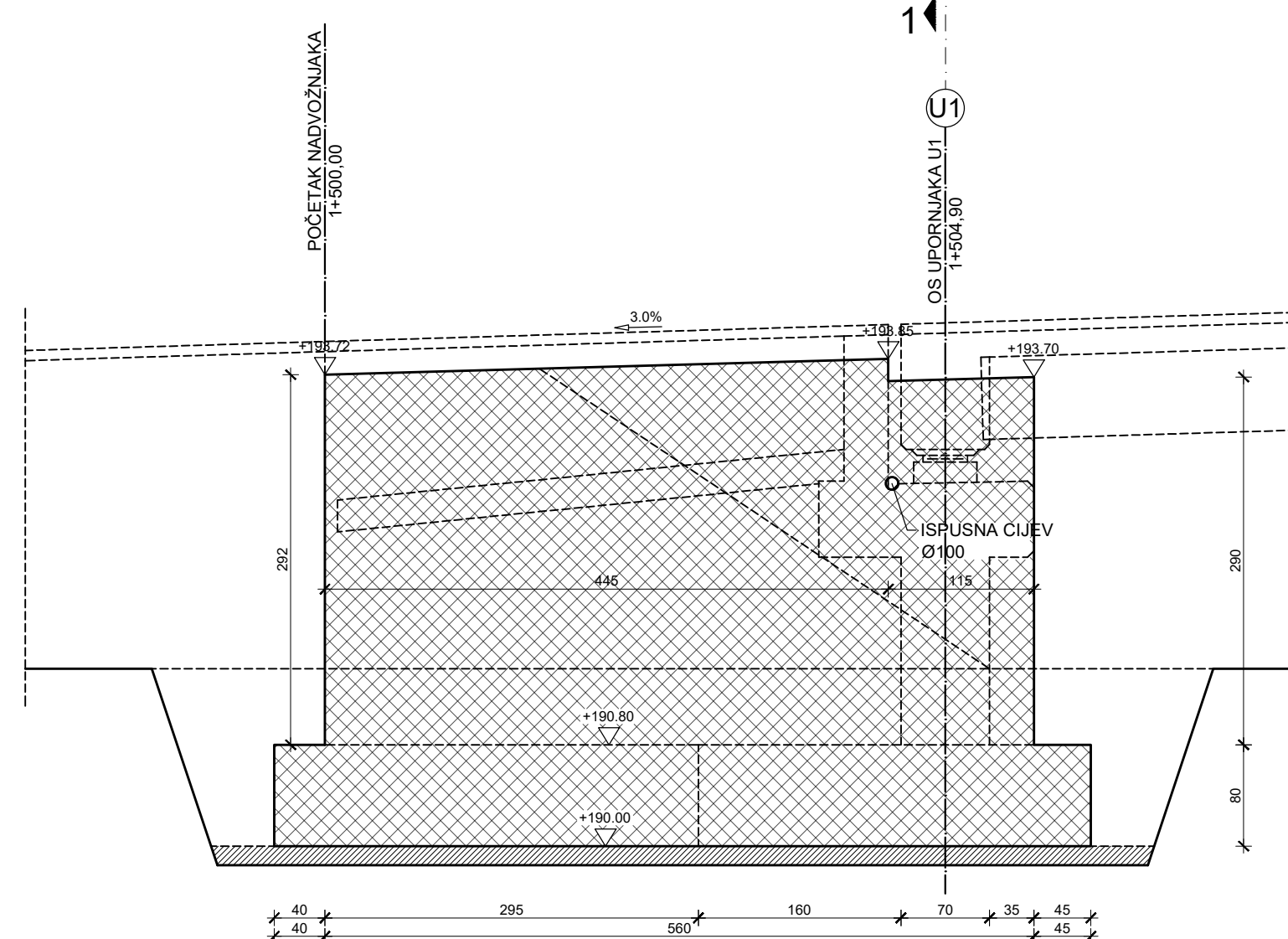
PRESJEK 6-6
