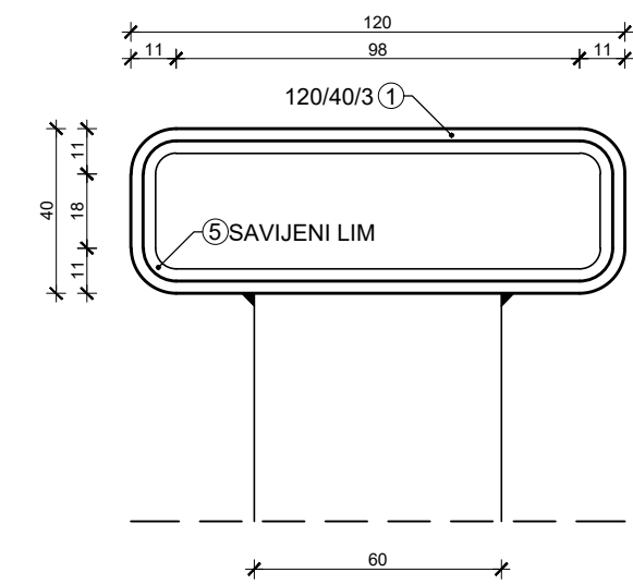
PRESJEK 2-2
