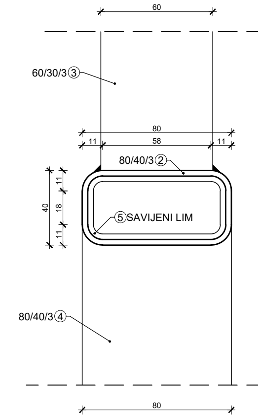
PRESJEK 3-3
