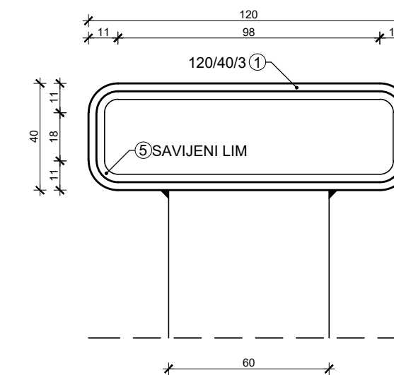
PRESJEK 2-2
