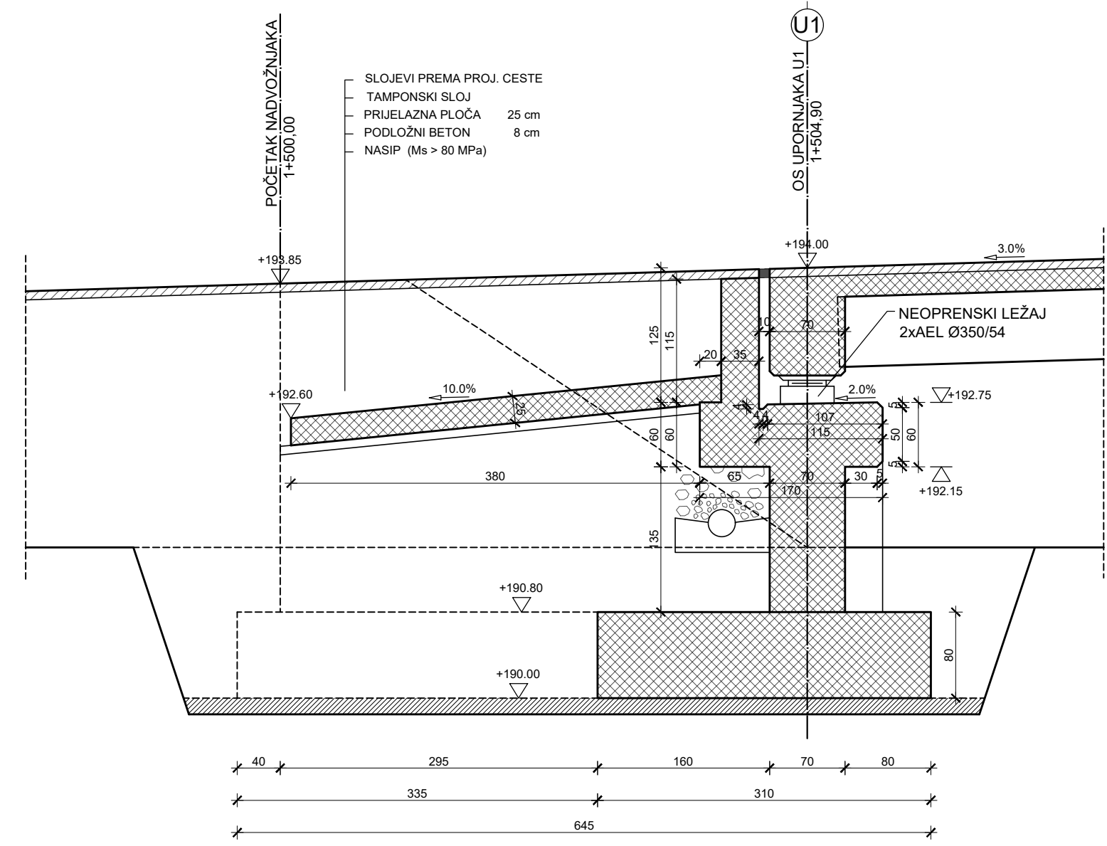
PRESJEK 2-2
