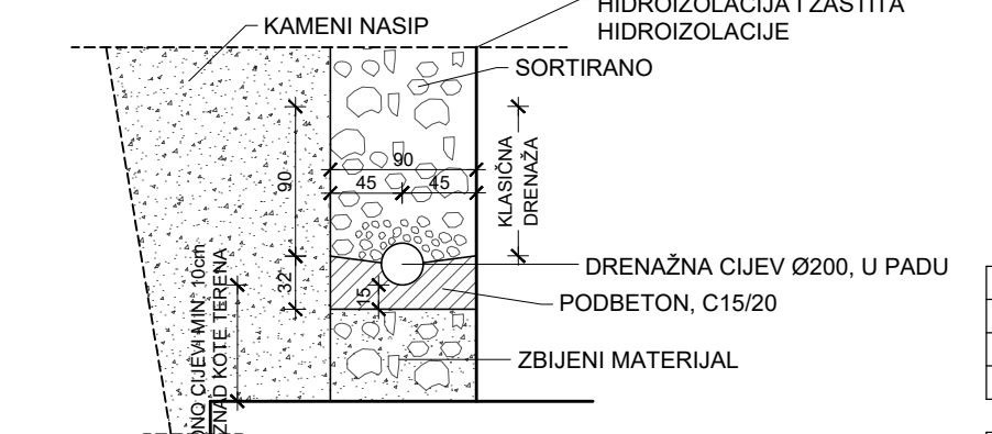
DETALJ DRENAŽE
