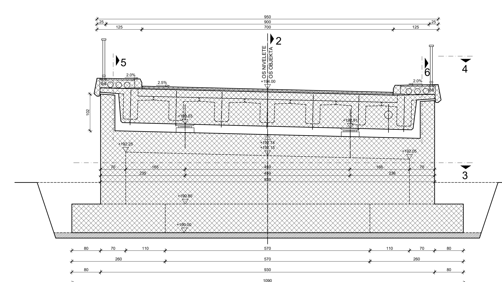
PRESJEK 1-1
