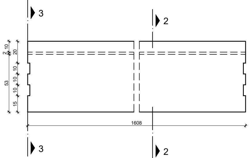
PRESJEK 1-1
