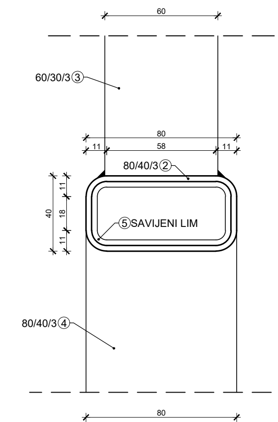
PRESJEK 3-3
