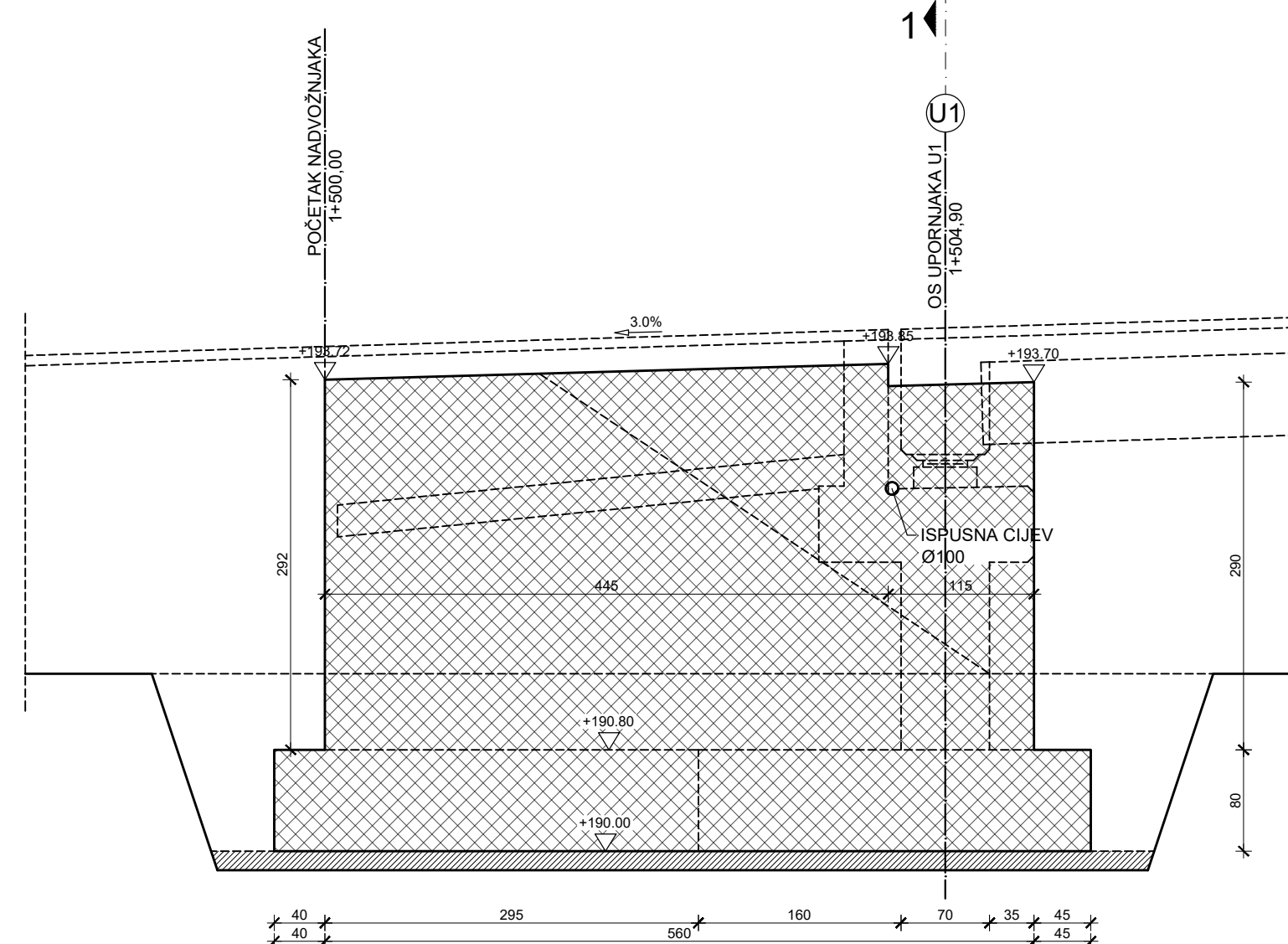
PRESJEK 6-6
