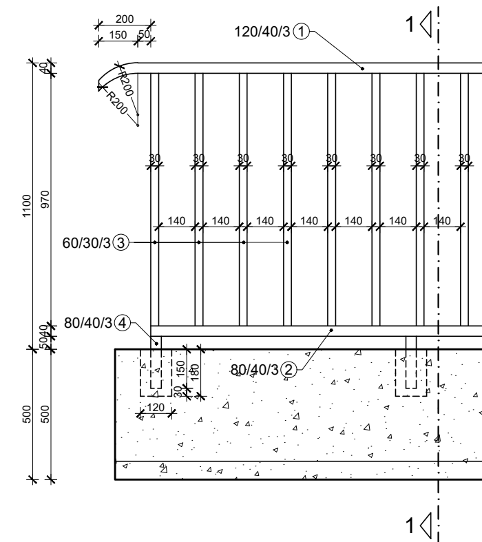
POGLED NA ELEMENT OGRADE M1:20
