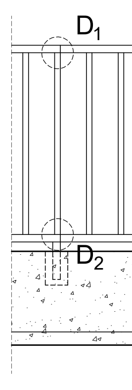
POGLED NA ELEMENT OGRADE M1:20
