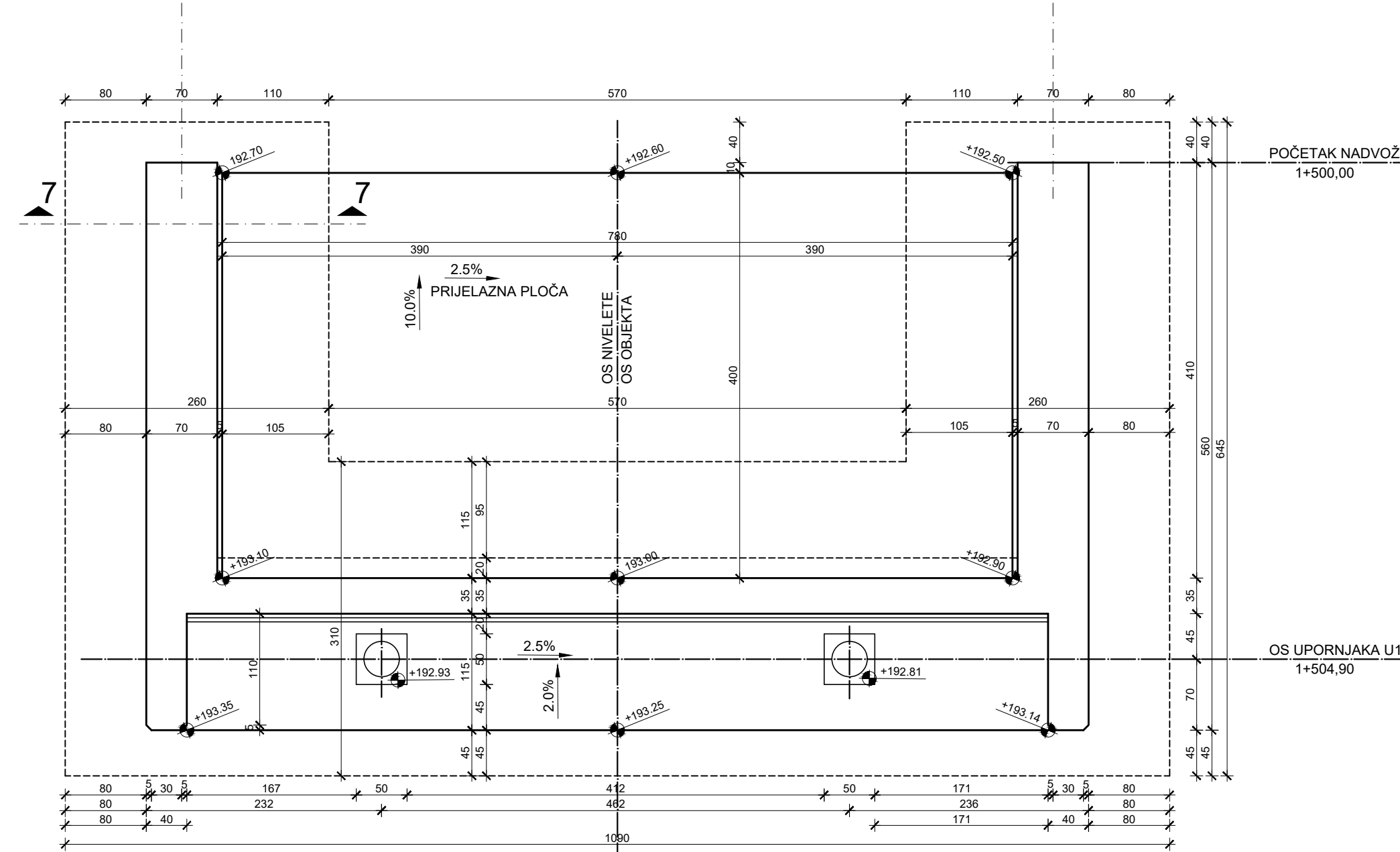
PRESJEK 4-4
