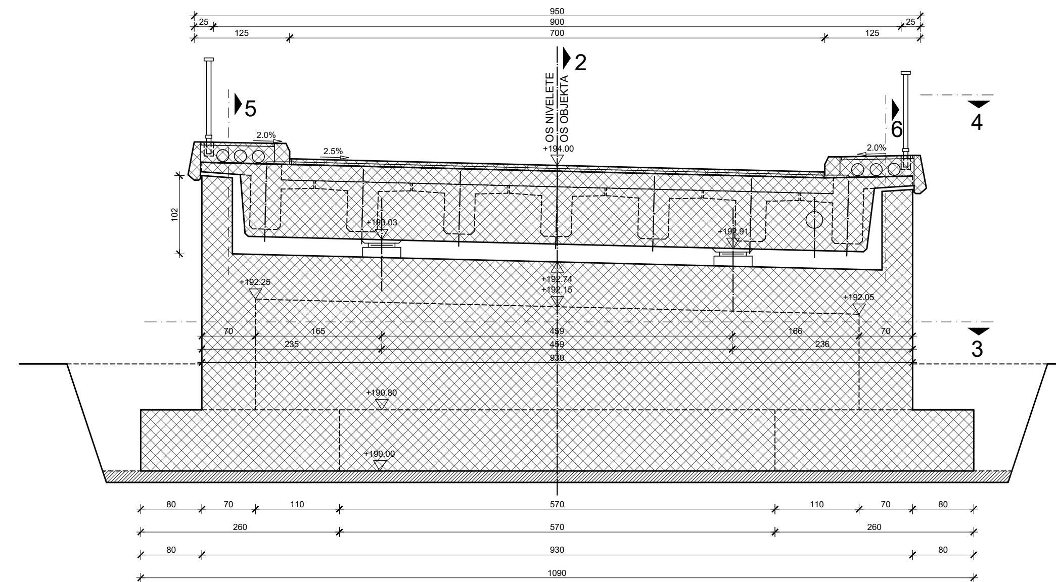
PRESJEK 1-1
