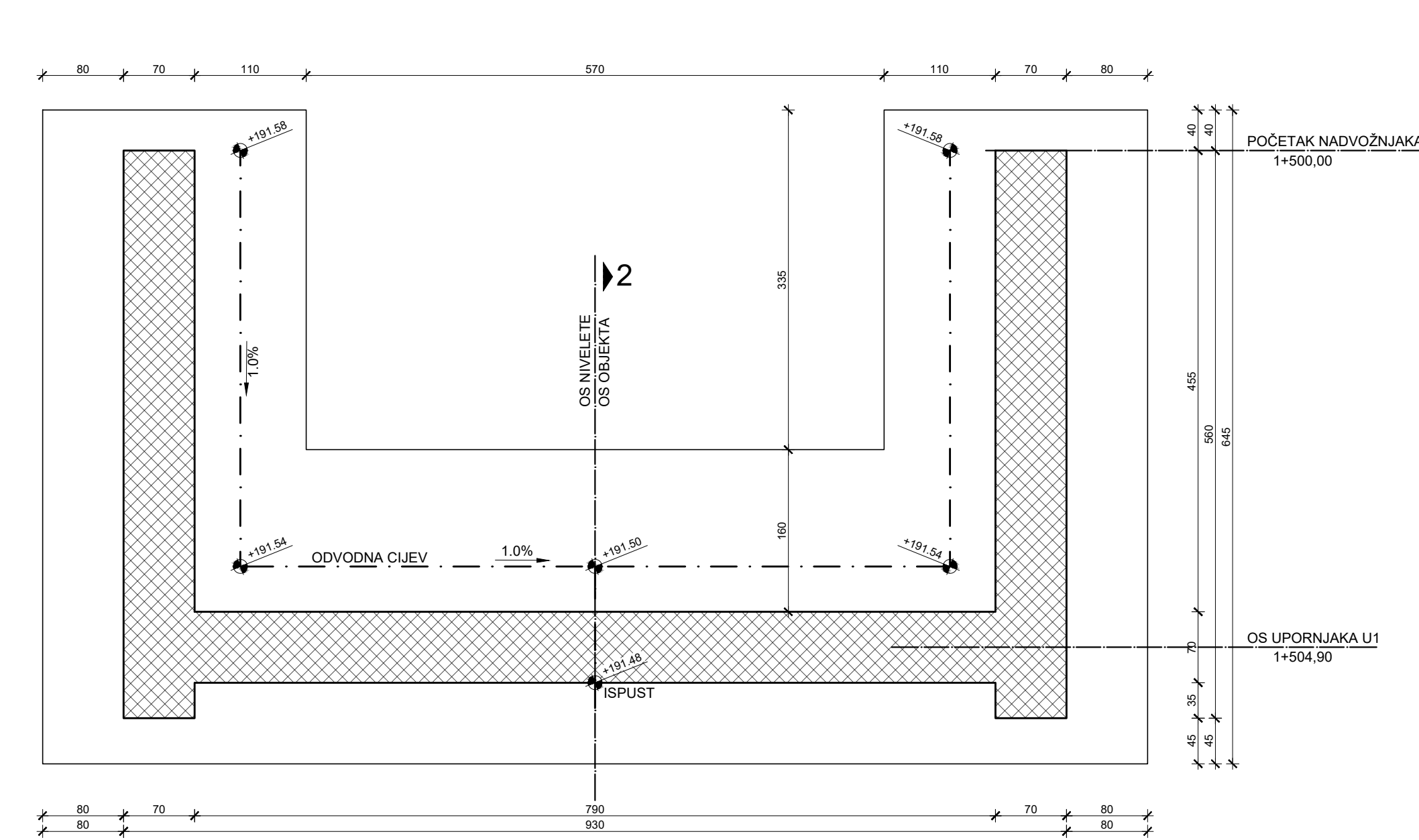
PRESJEK 3-3
