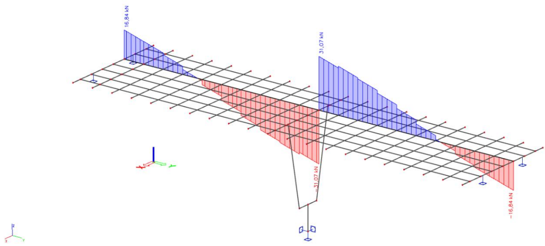
Slika 12. Dodatno stalno opterećenje-poprečne sile ( V_z ) u kN
