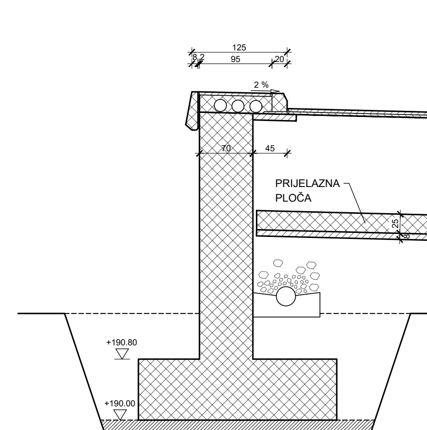
PRESJEK 7-7
