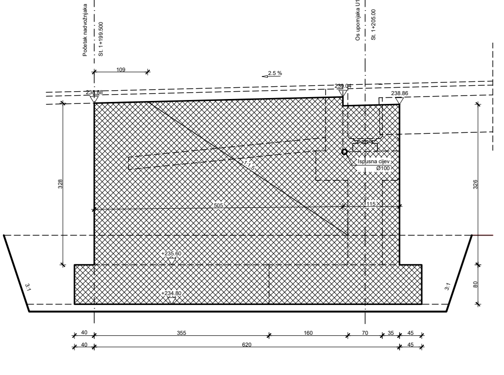
Presjek 6-6
