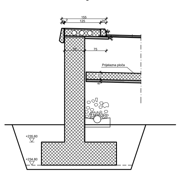
Presjek 7-7
