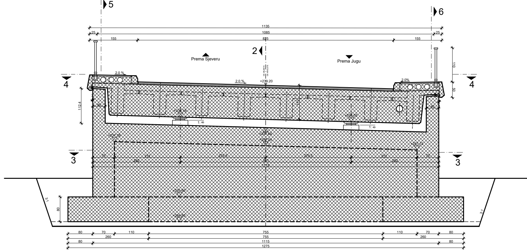
Presjek 1-1
