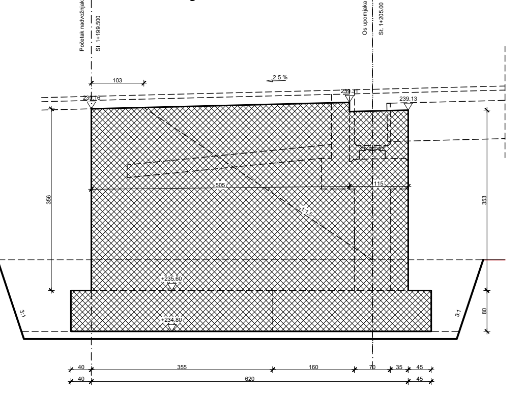
Presjek 5-5
