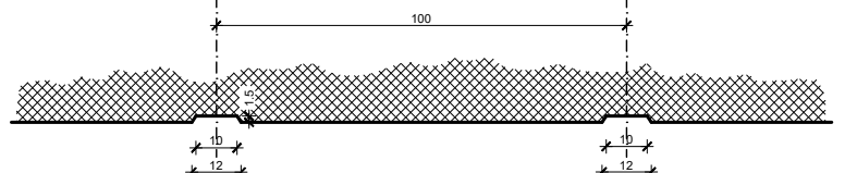
Detalj kanelura
