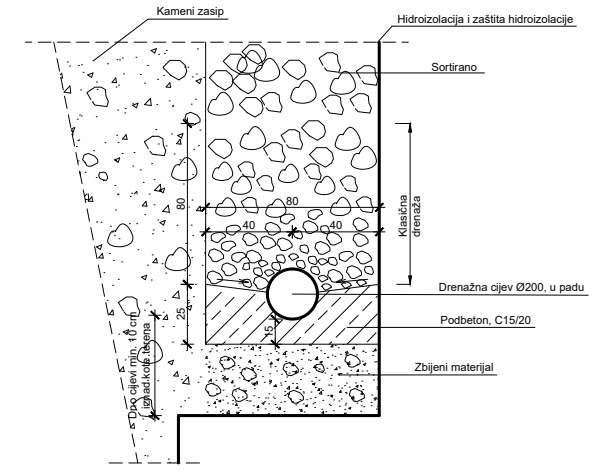
Detalj drenáže
