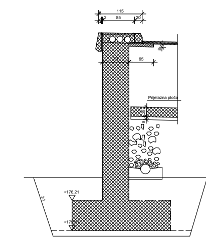
Presjek 7-7
