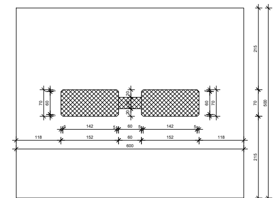
Presjek 4-4
