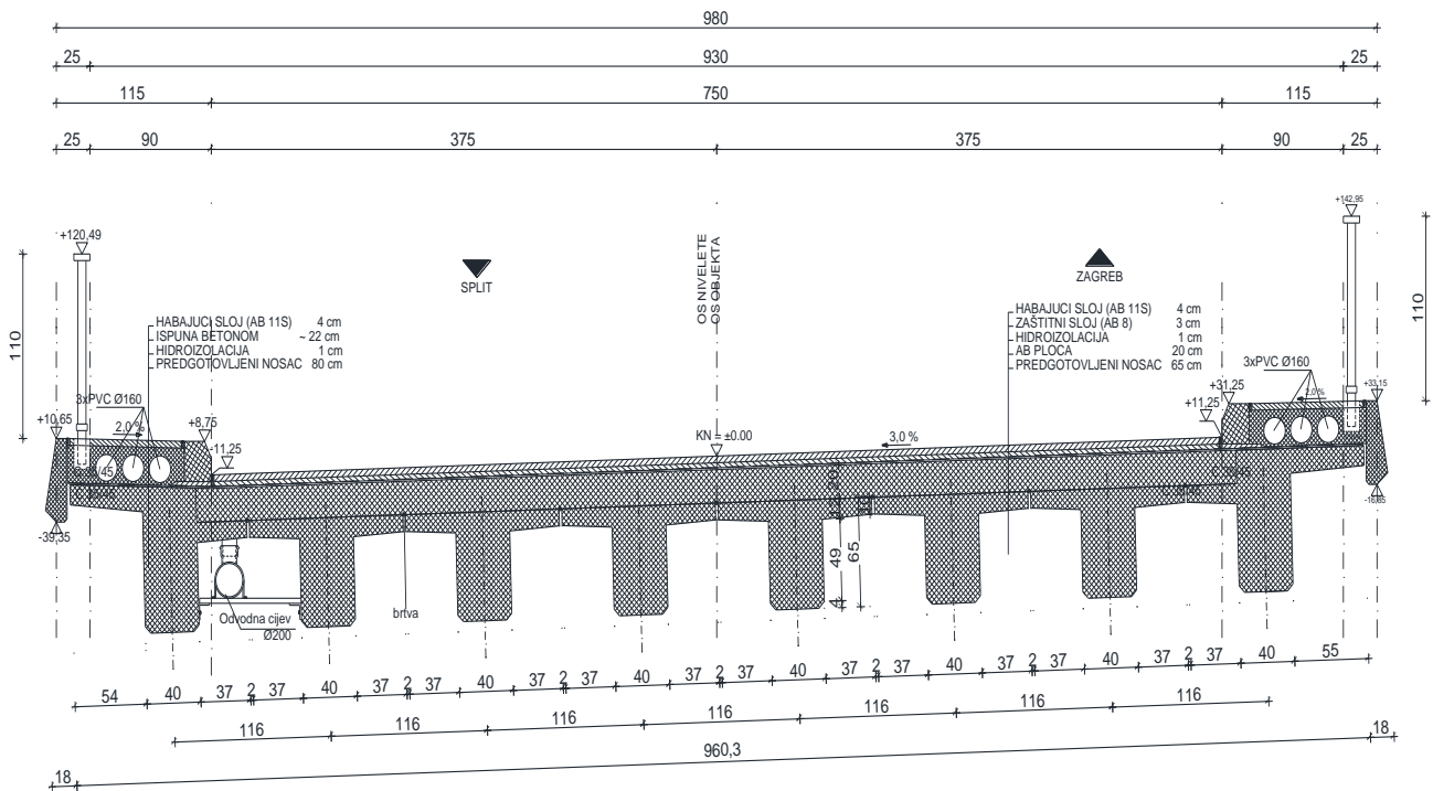
Slika 1. Poprečna dispozicija mosta
