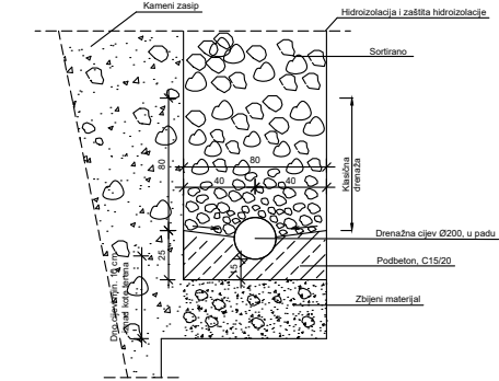
Detalj drenaže
