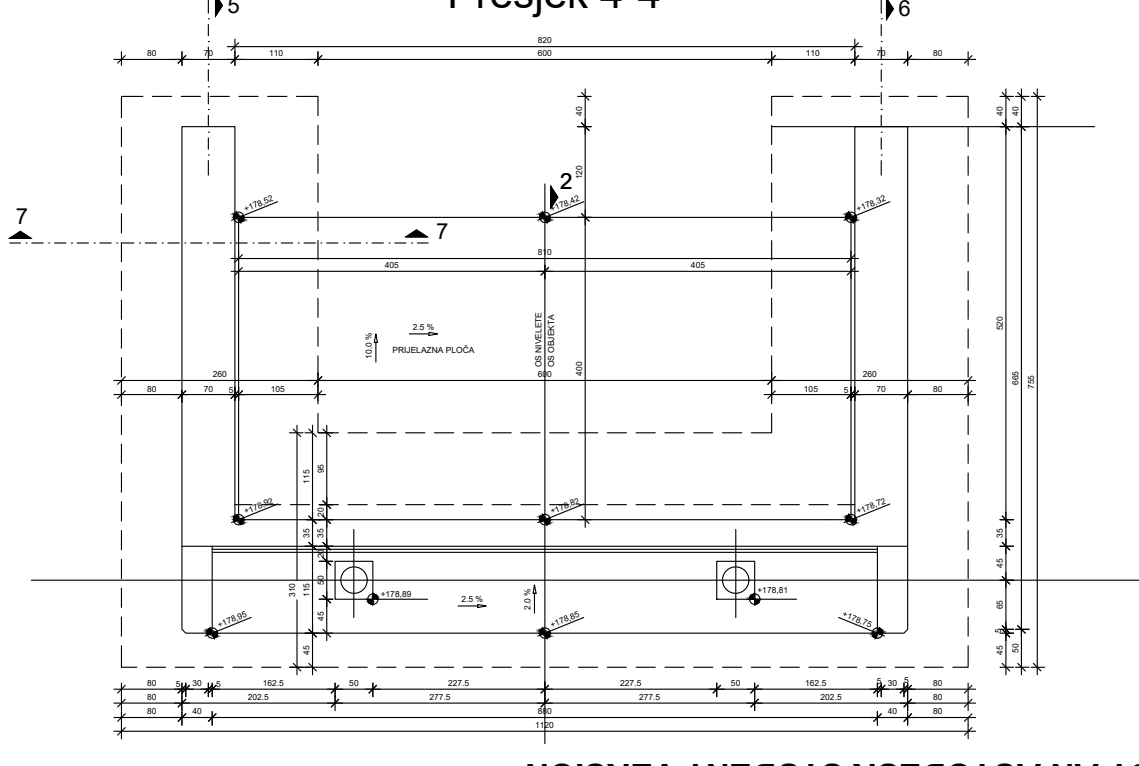
Presjek 4-4
