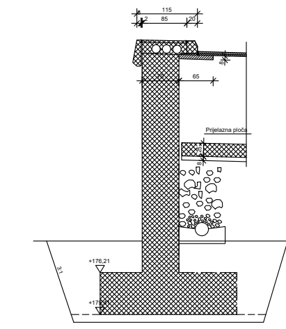
Presjek 7-7
