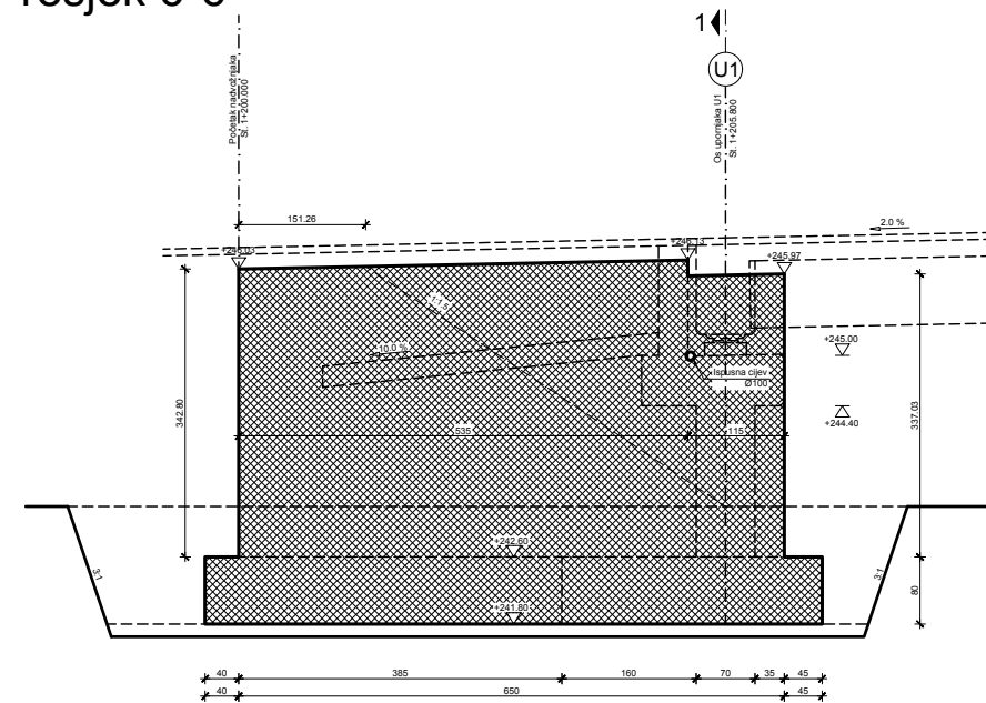
Presjek 6-6
