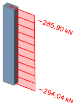
Slika 13.16. prikaz N
