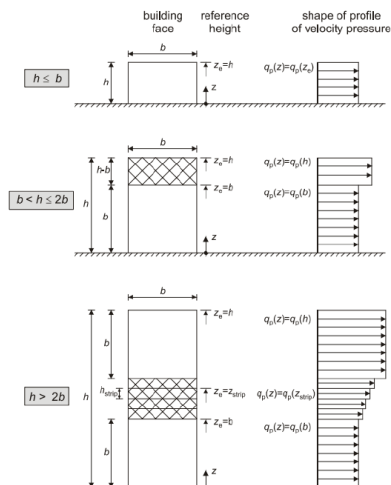
Slika 8.7. Određivanje koeficijenta vanjskog tlaka vjetra
