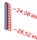
Slika 13.46. prikaz N_{prip}
