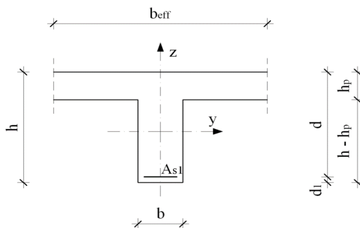
Slika 12.11 – Poprečni presjek grede u polju
