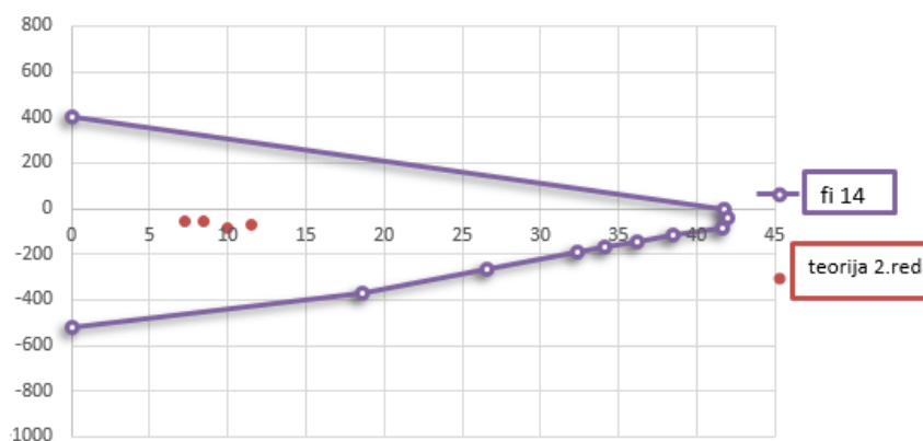
Slika 13.63. Dijagram interakcije
