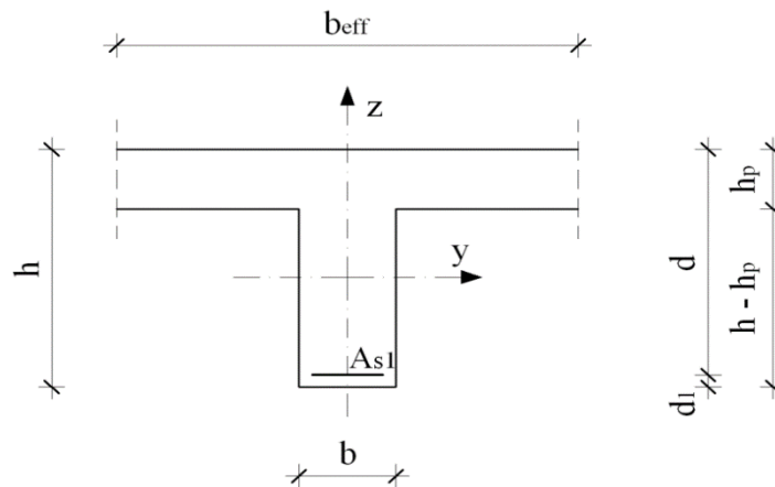
Slika 12.25. – Poprečni presjek grede u polju
