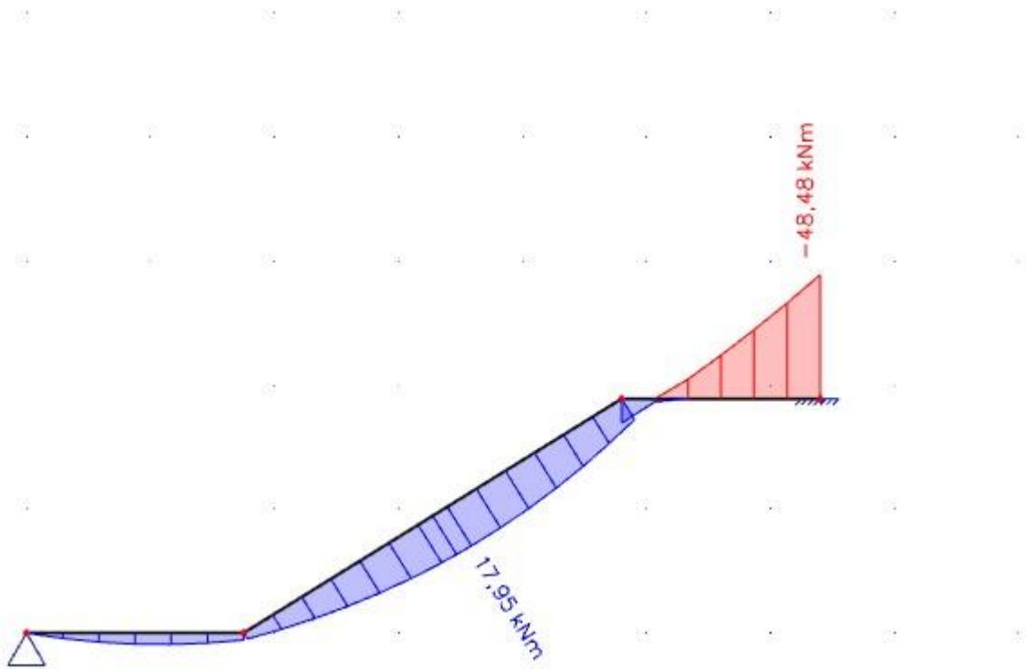
Slika 10.1 Moment savijanja na stubištu
