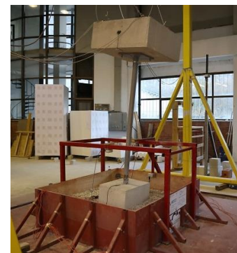
f) M_4 on layer h_p = 0.3 m
