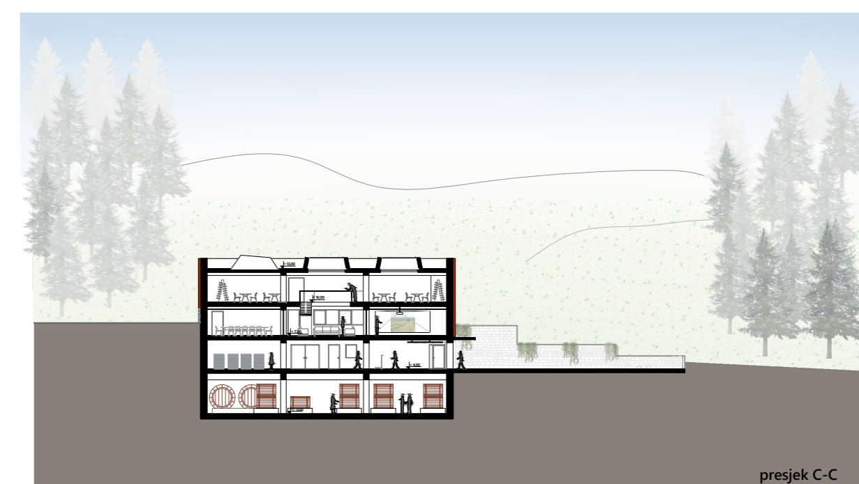
presjek C-C
