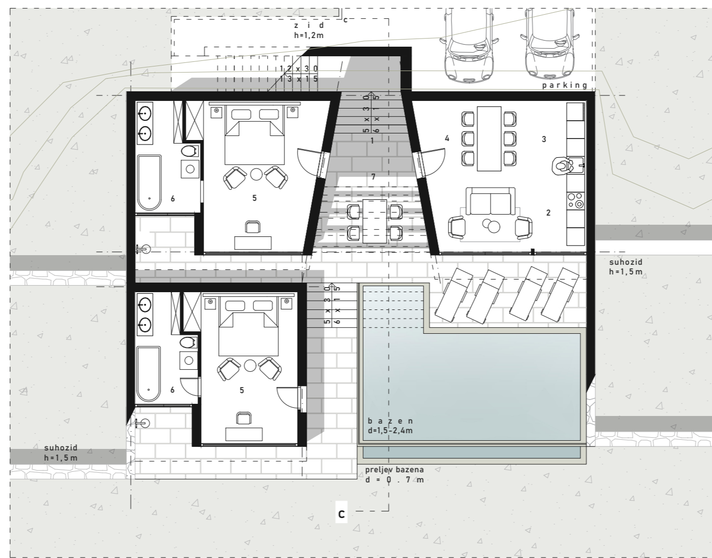
TLOCRT VILE
