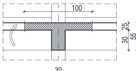
Slika 12.24. Poprečni presjek gređe u polju
