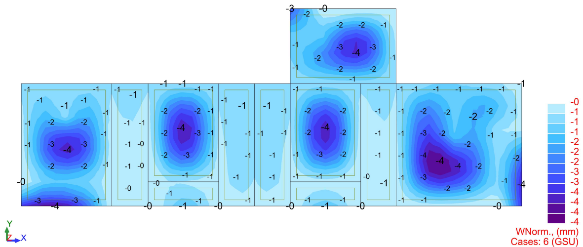
Slika 10.55. Prikaz progiba U_z [mm]
