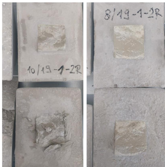
Slika 39. Uzorci 10/19 i 08/19 imobilizirani mortom recepture 2
