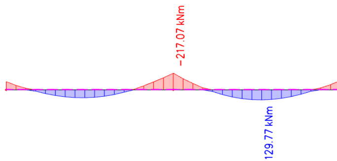
Slika 4.7. Dijagram momenata savijanja M_y na gredi(GSN)
