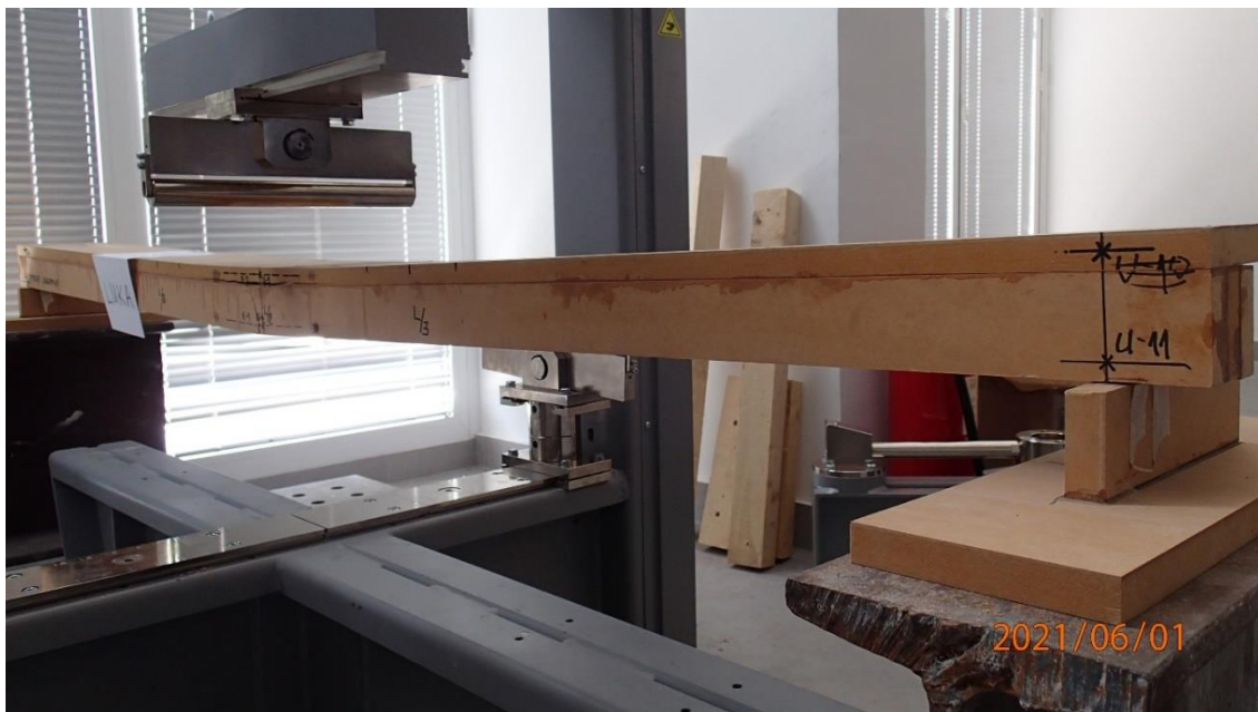
Slika 63: Slom nosača
