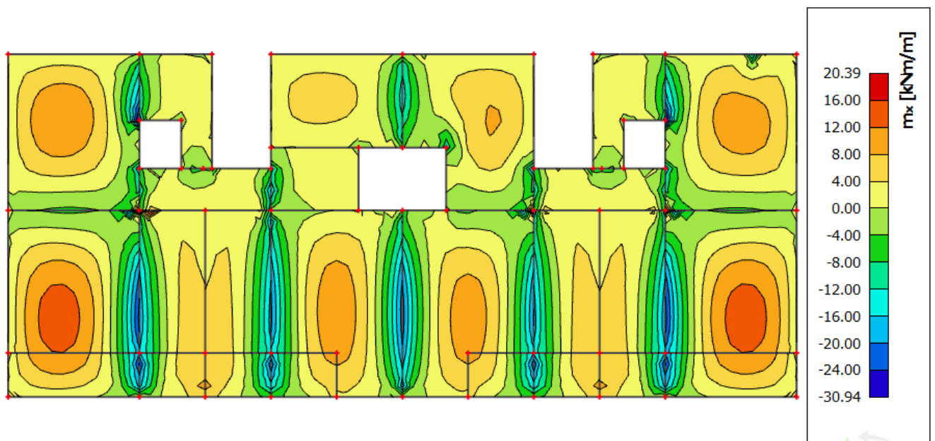
Slika 7.19 Moment savijanja M_{Ed,x} ( \text{kNm/m} ) za GSU-1
