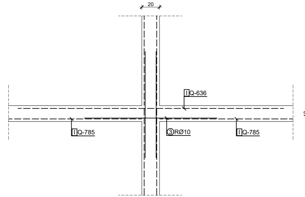
Presjke 2-2 M 1:25
