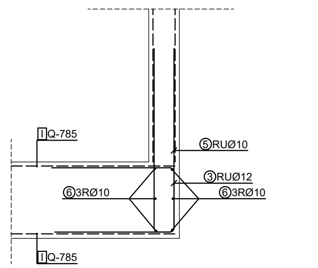
Presjke 2-2 M 1:25
