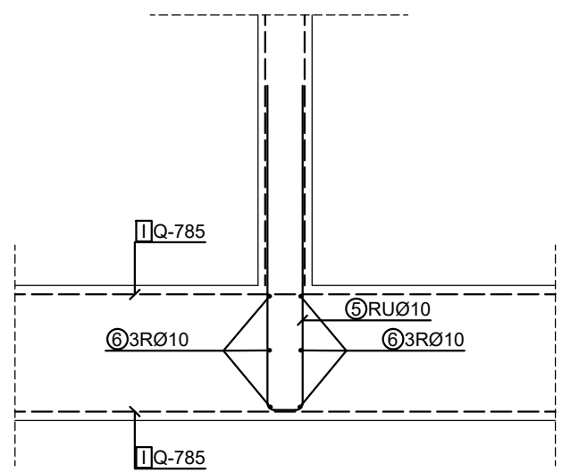
Presjke 2-2 M 1:25
