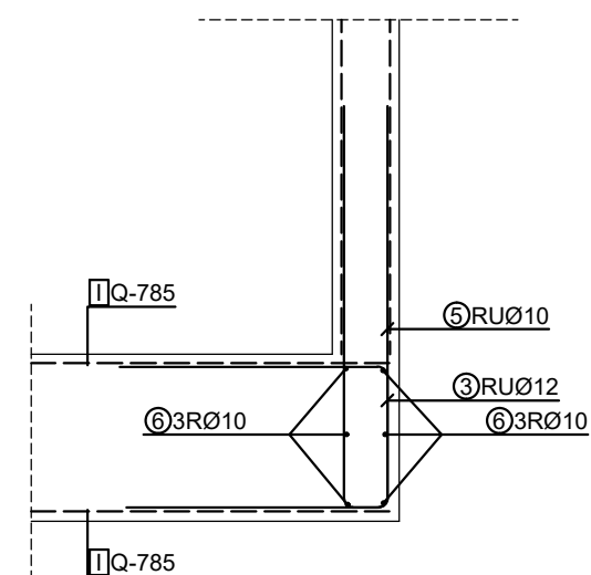
Presjke 2-2 M 1:25
