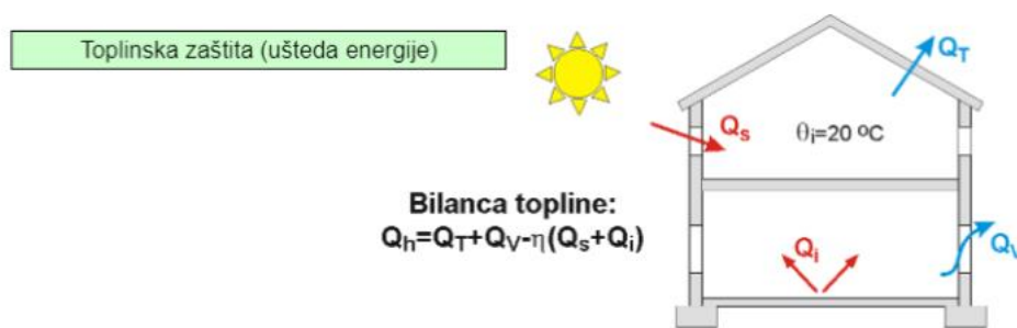
Slika 95. Bilanca topline
