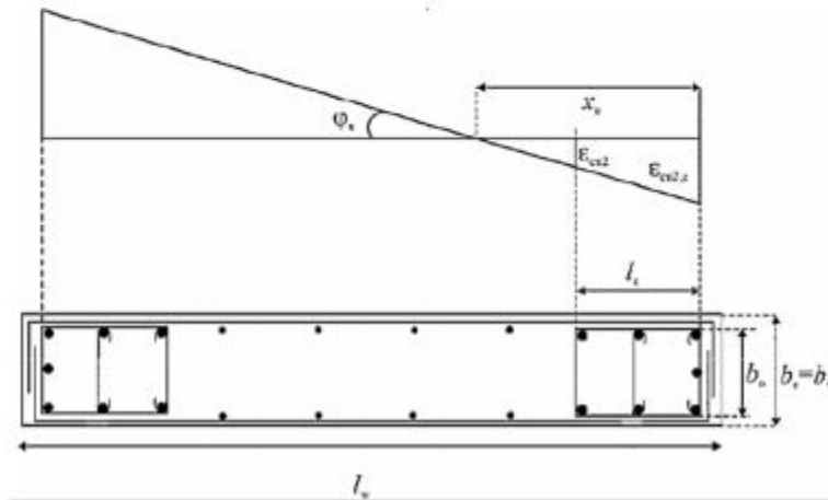
Slika 88. Shema potresne armature
