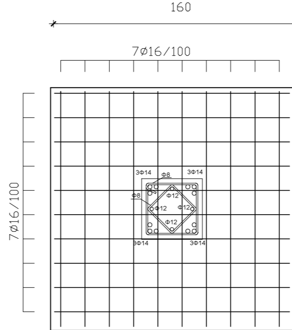
Presjek 2-2 M 1:25
