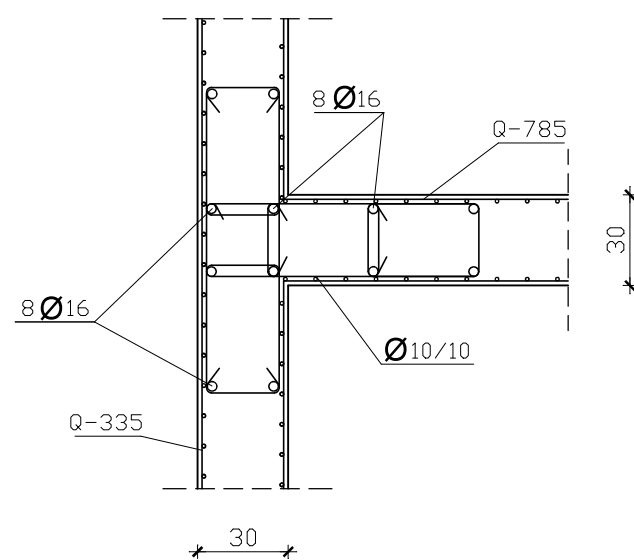
Detalj Z4
