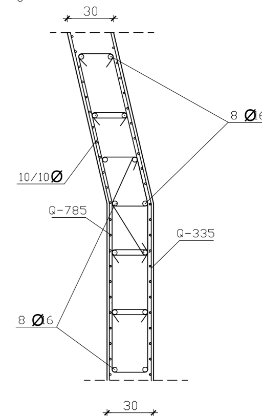
Detalj Z3
