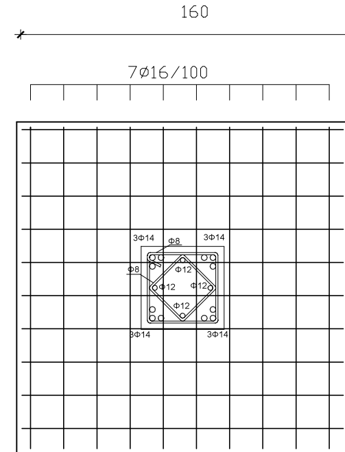
Presjek 2-2 M 1:25
