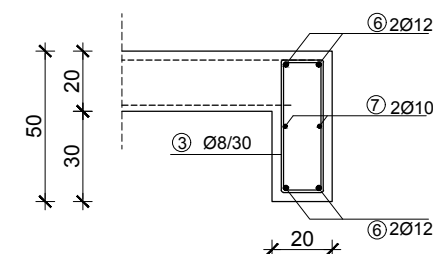
PRESJEK 3-3
