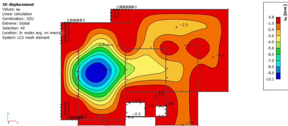
Slika 65. Maksimalni progib ploče POZ 100
