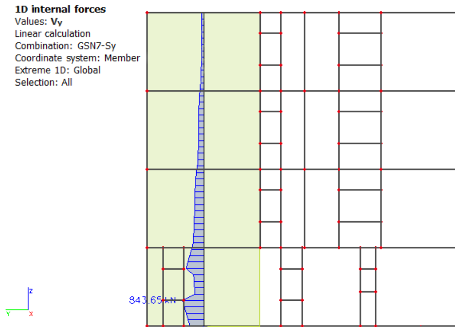
Slika 146. Poprečne sile u zidu Zy1 (kN)
