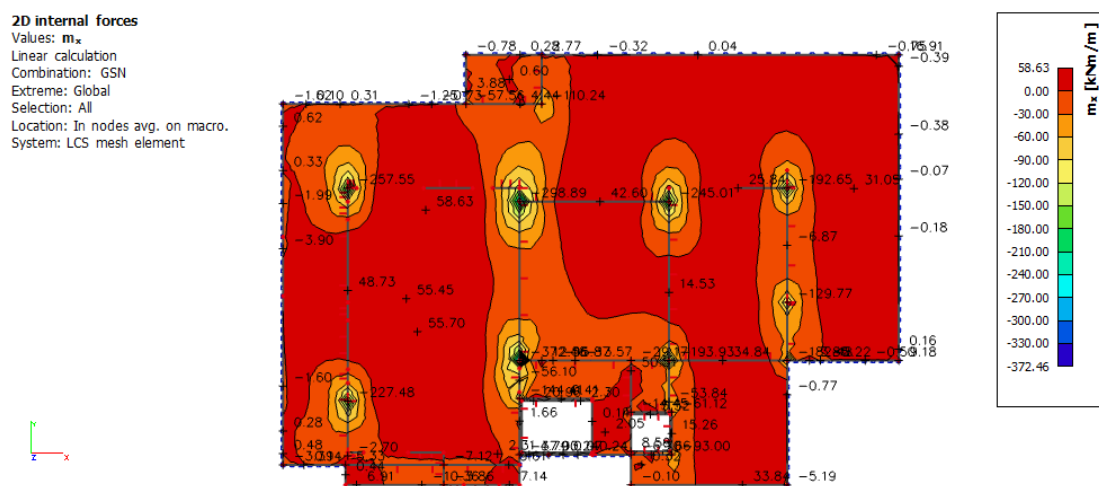
Slika 60. Moment savijanja M_x ploče POZ 100 (kNm)
