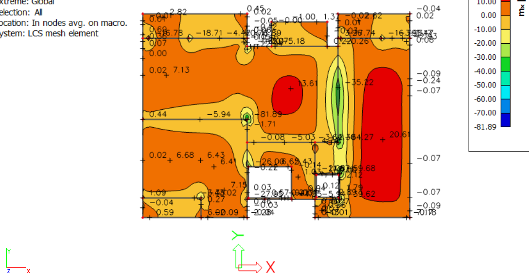
Slika 38. Moment savijanja GSU M_x ploče POZ 500 (kNm)
