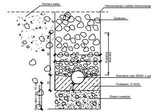
Detalj drenaže
