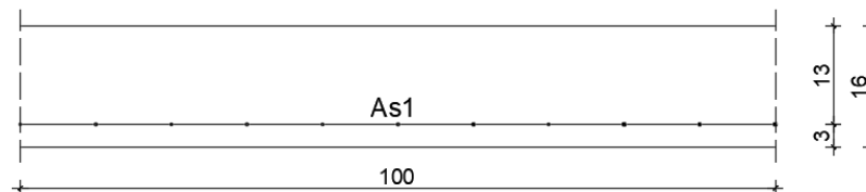
Slika 105. Skica armature ploče u polju
