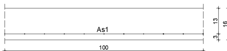
Slika 131. Skica armature ploče u polju
