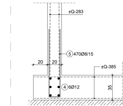
PRESJEK 1-1 M 1:25
