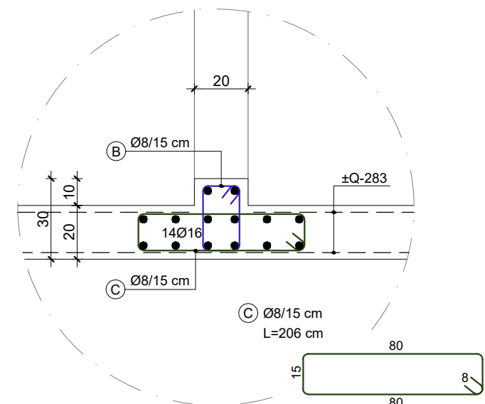
Detalj C
