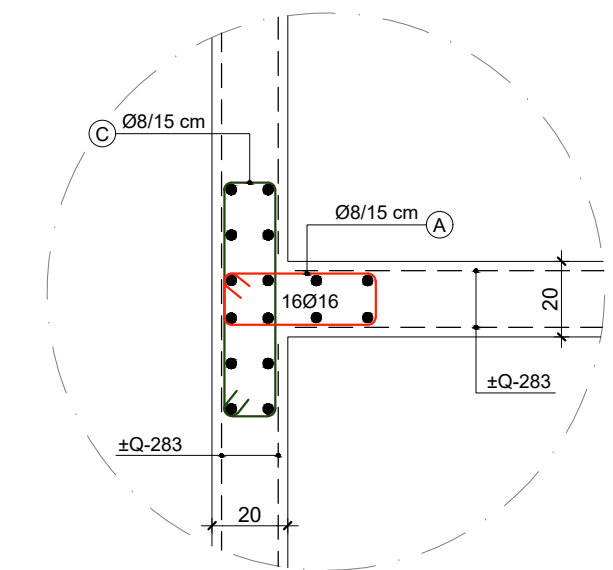
Detalj D
