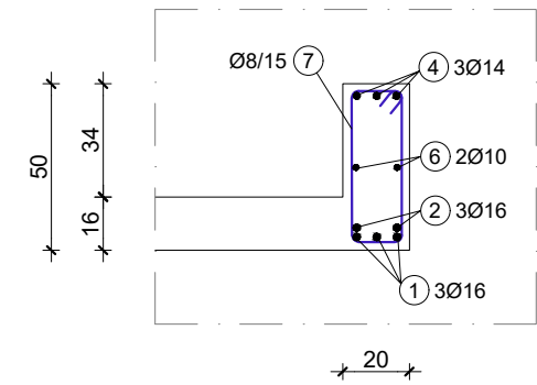
PRESJEK A-A M 1:25
