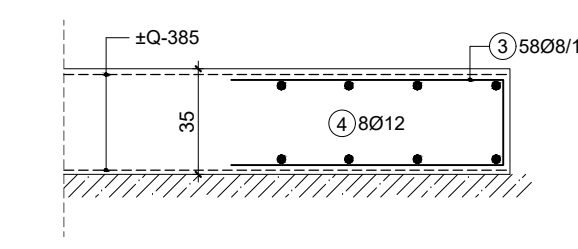
PRESJEK 2-2 M 1:25
