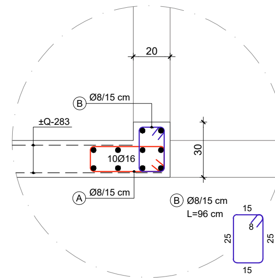
Detalj B
