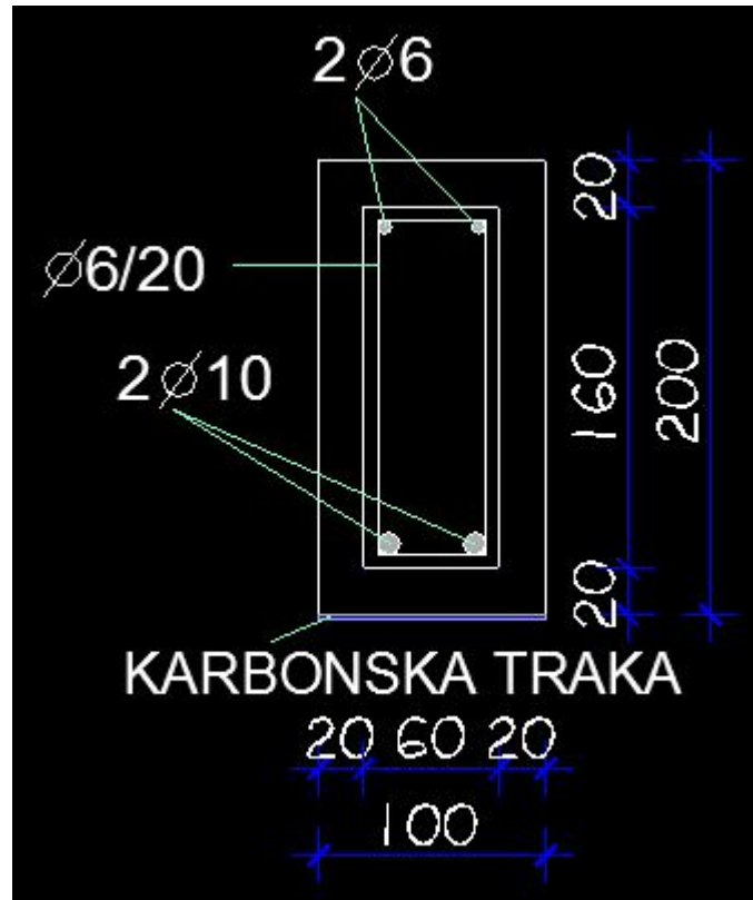
Crtež 1.3: Poprečni presjek grede G2
