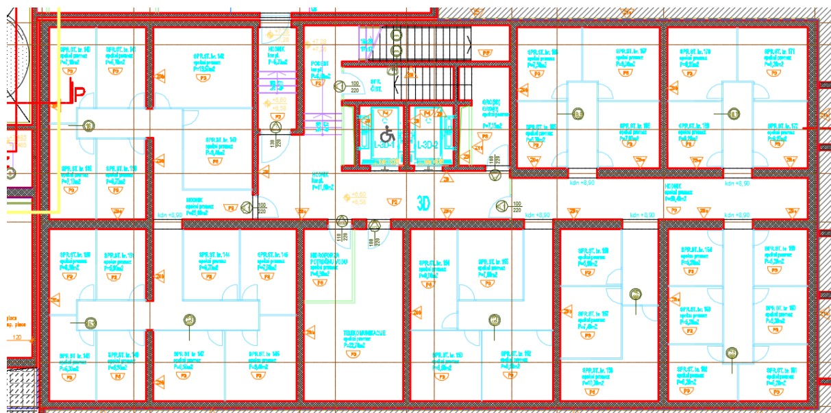
Slika 2.3. Tlocrt podruma -2
