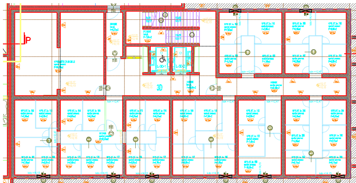
Slika 2.4. Tlocrt podruma -1
