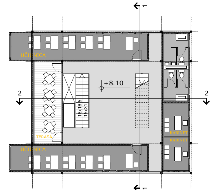
TLOCRT 3. KATA
