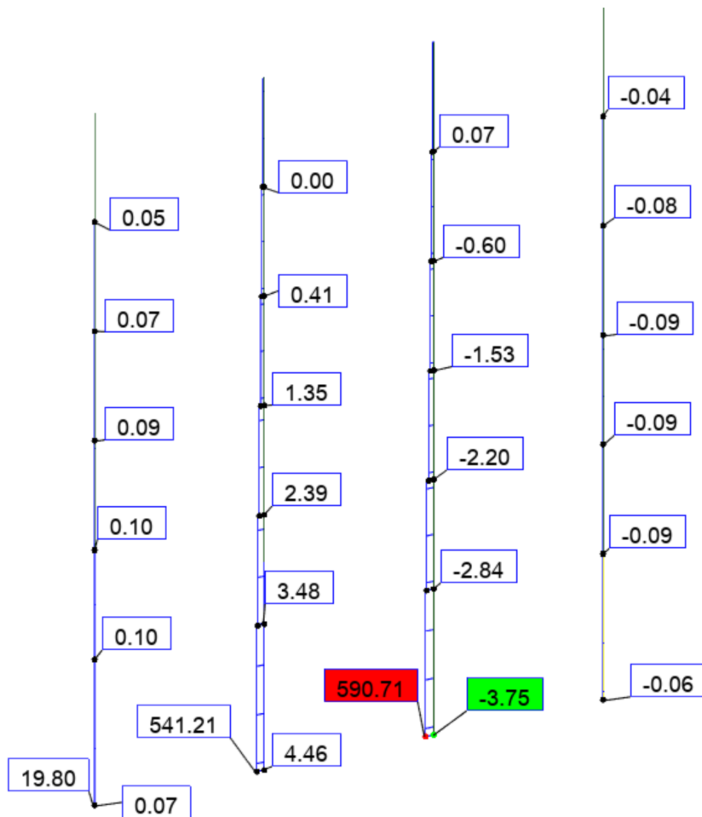
Slika 7.4. Uzdužne sile
