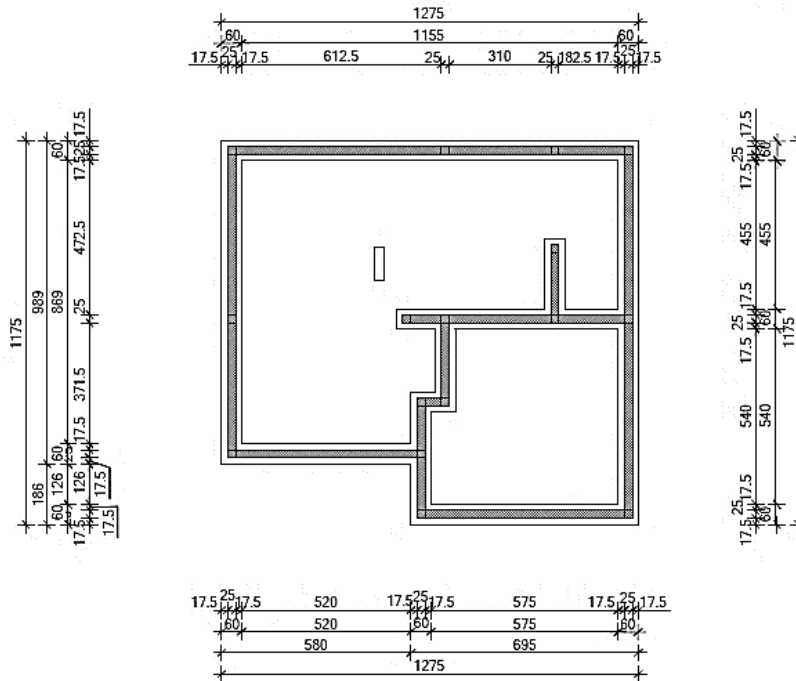
Slika 18. Tlocrt temelja
