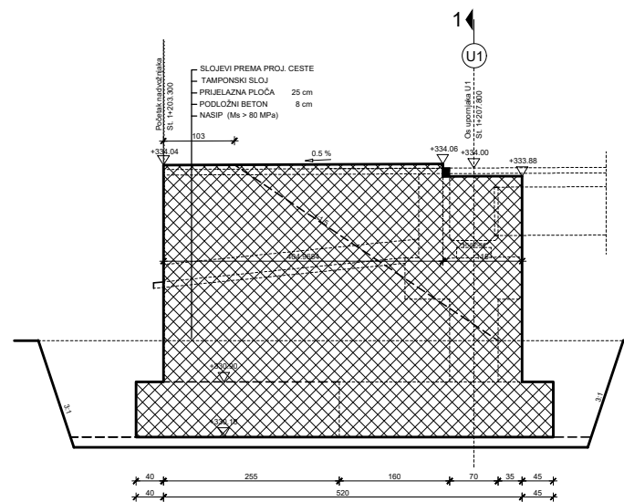
Presjek 5-5
