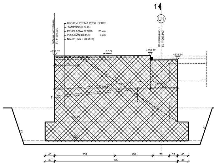
Presjek 6-6
