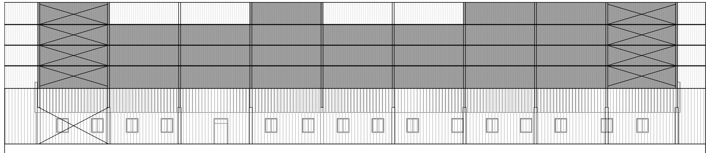
JUŽNO PROČELJE
