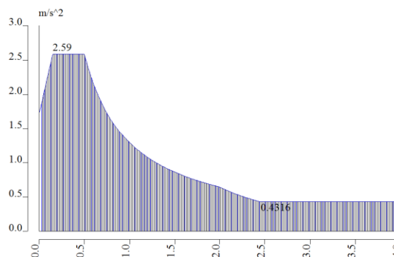
Računski spektar odgovora za oba smjera (X, Y) za a_{gr,GSN}=0.22 \text{ g} = 2.15 \text{ m/s}^2 , q=2.5 , tlo B
