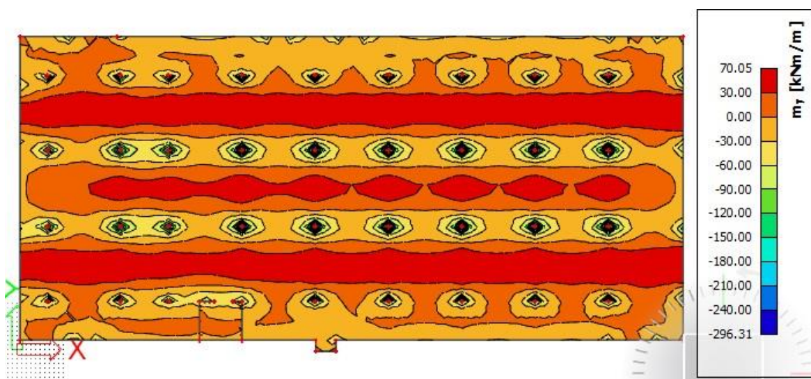
Slika 6.1.2.3 Moment savijanja M_{Ed,y} ( \text{kNm/m} ) za GSU-1
