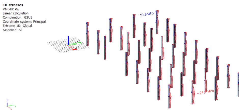
Slika 9.2 Srednje tlačno naprezanje u stupovima \sigma_{c,Ed} (MPa) za GSU-1
