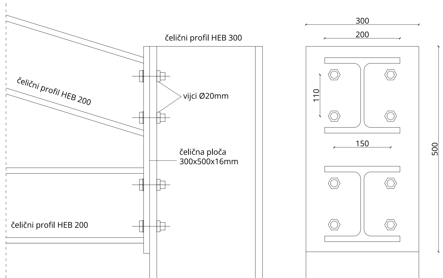
3. spoj HEB 300 čeličnog stupa i čelične rešetke
