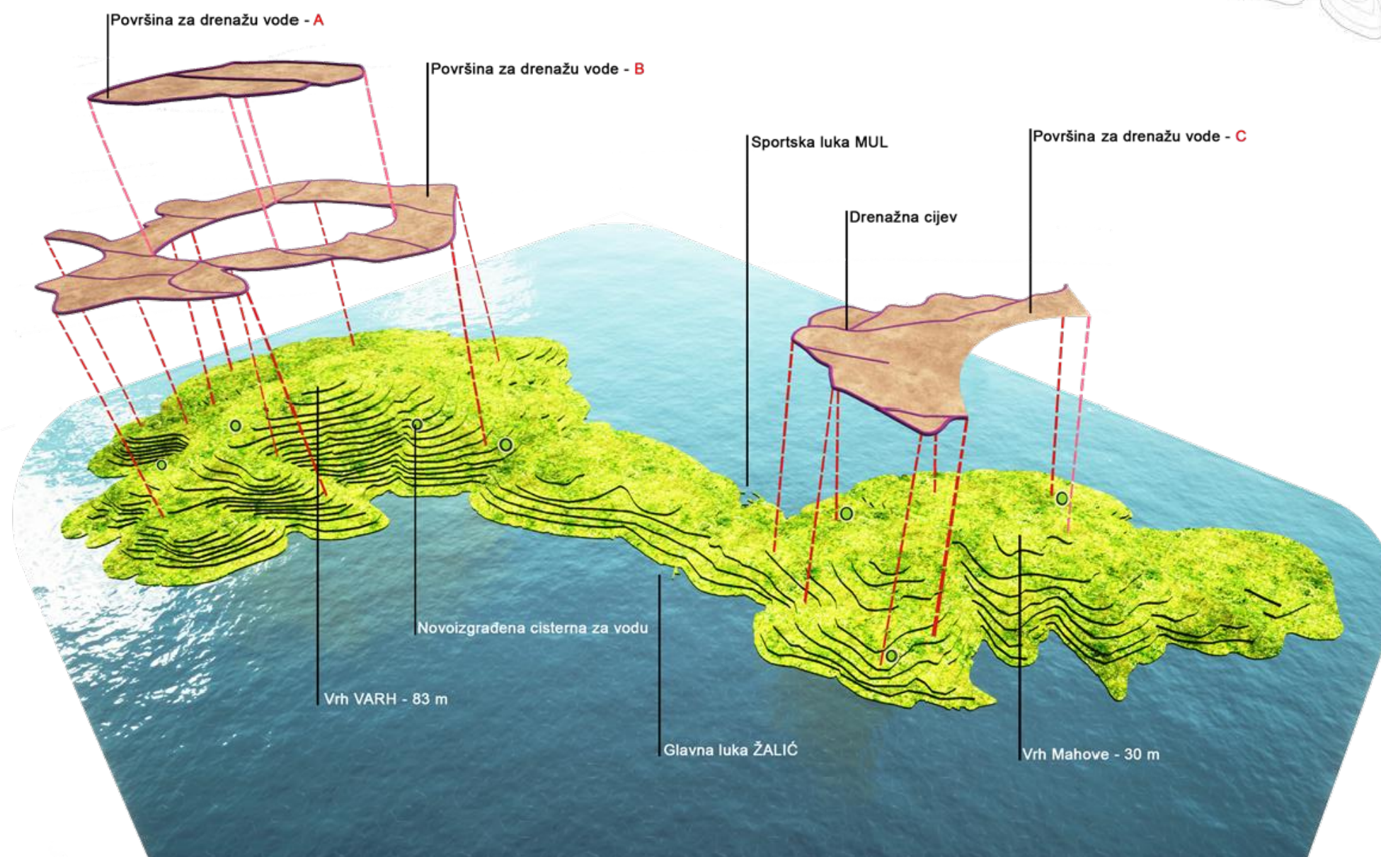
Slika 40. - Smještaj sustava na otoku - 3D Slika 41. - Smještaj sustava na otoku - 2D
